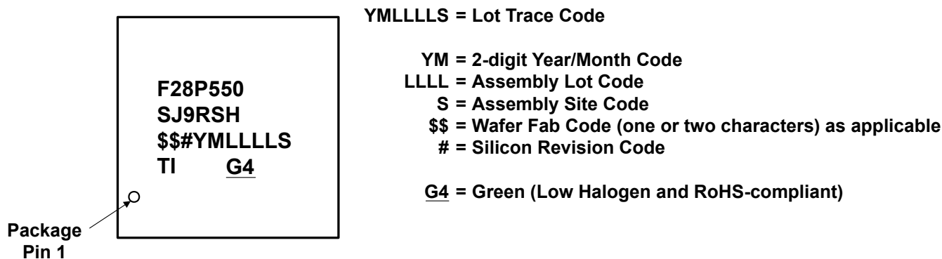
図 10-9. RSH パッケージのパッケージ マーキング – 車載以外
