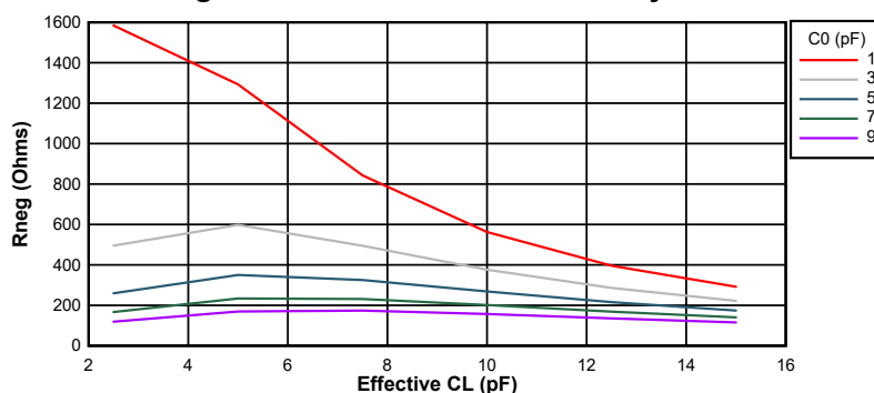
図 6-17. 20MHz 時の負性抵抗変動
