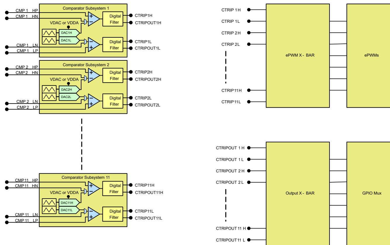
図 6-63. CMPSS の接続
