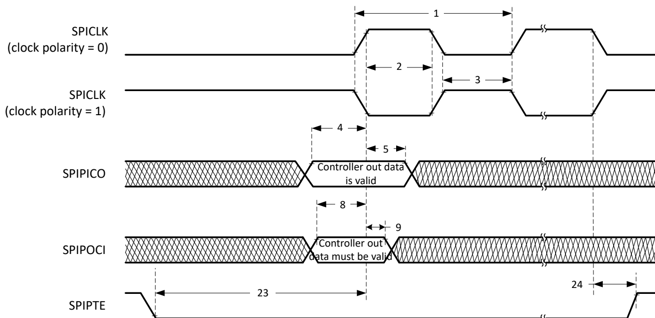
図 6-99. SPI コントローラ・モードの外部タイミング (クロック位相 = 0)
