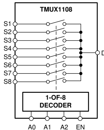
図 7-11. TMUX1108 Functional Block Diagram
