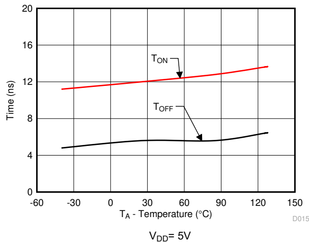
図 6-15. T_{ON} (EN) and T_{OFF} (EN) vs Temperature
