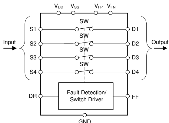
ブロック図
