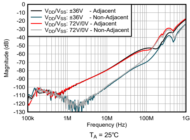
図 6-25. クロストークと周波数との関係
