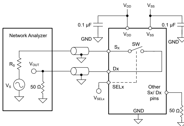
図 7-6. オフ絶縁測定時の設定
