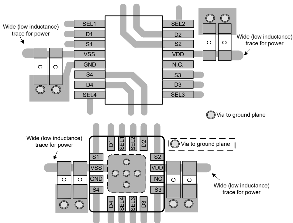
図 8-5. TMUXL5412 レイアウト例
