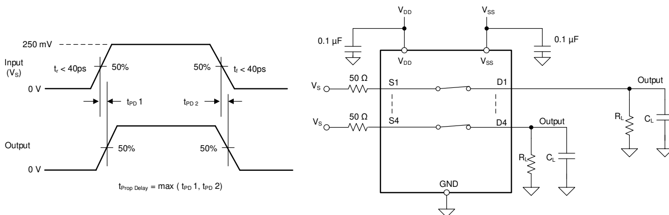
図 6-5. 伝搬遅延測定時の構成
