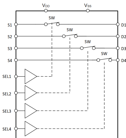
TMUXL5412 ブロック図
