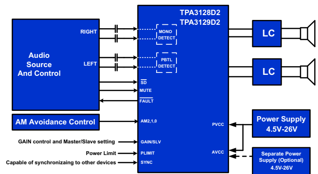
アプリケーションの簡略回路図
