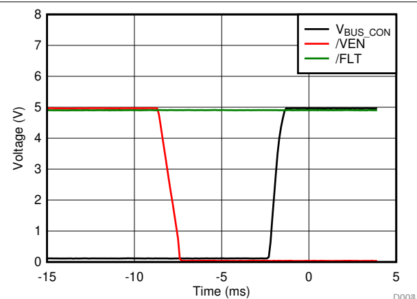
图 6-4. V_{BUS} t_{ON} Time
