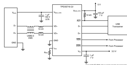
代表的なアプリケーション回路図
