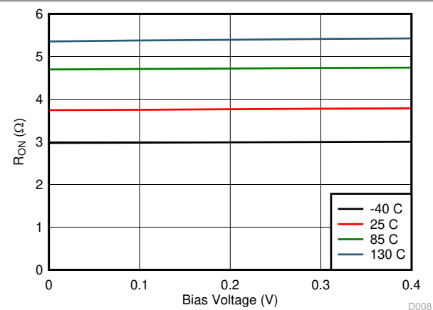
图 6-6. Data Switch R_{ON} vs Bias Voltage
