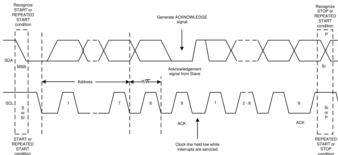
图 7-5. I 2 C Bus Protocol
