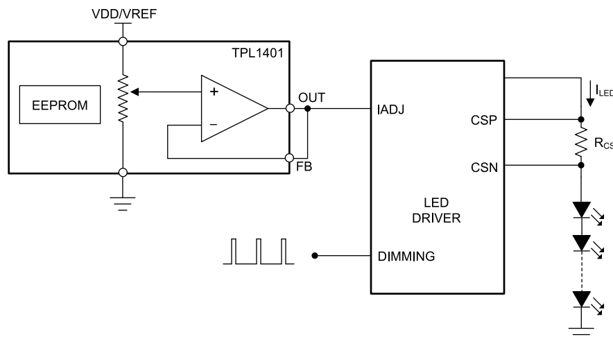
図 8-1. Programmable Current Limit
