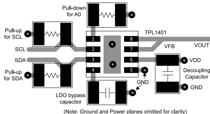
✎ 10-1. Layout Example
