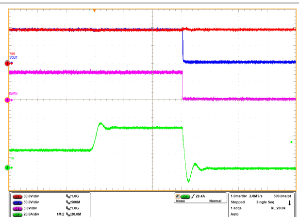
図 8-9. 過電流保護
