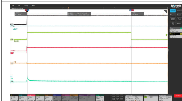
図 6-25. 過渡過電流ブランキング
