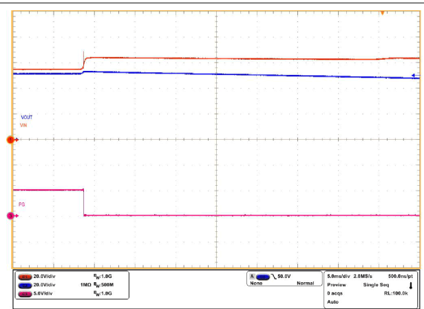
図 8-7. 過電圧保護
