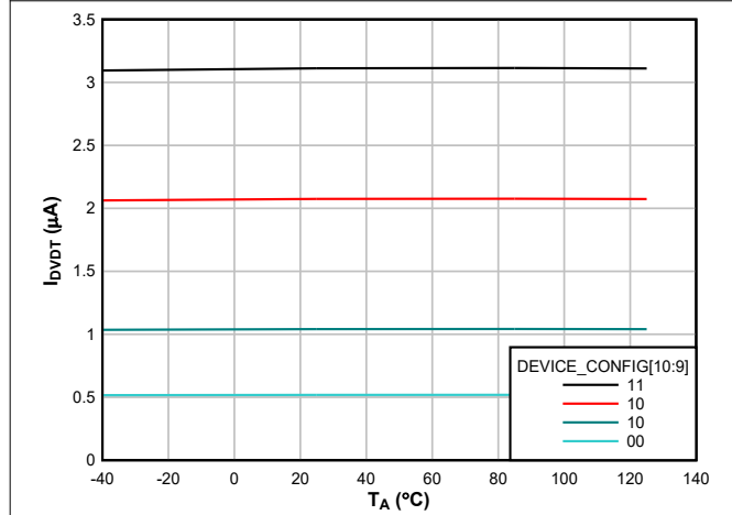
図 6-15. 温度範囲にわたる DVDT ピン充電電流
