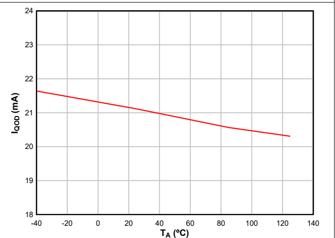
図 6-18. 温度範囲にわたる QOD シンク電流
