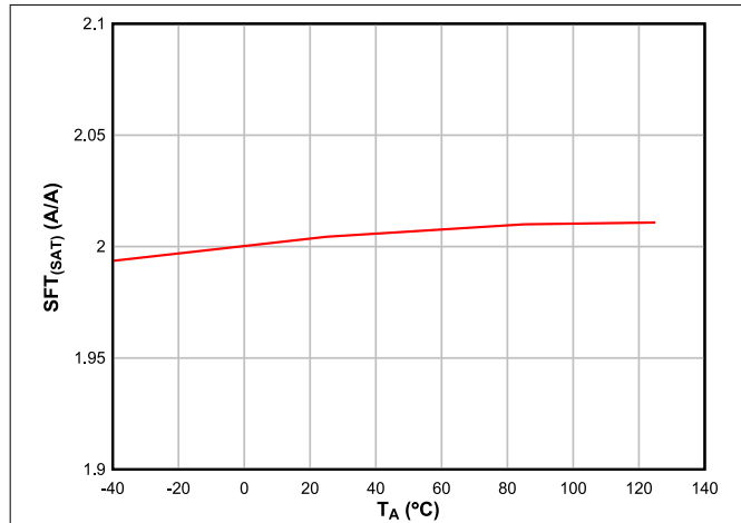
図 6-13. 温度範囲にわたる起動時のスケラブルな高速トリップスレッシュホルド比
