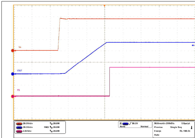
図 8-6. VIN は 0V から 54V に上昇
