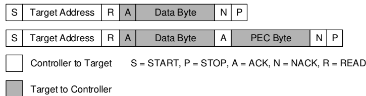
図 7-9. 受信バイト
