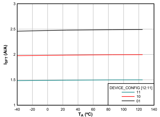
図 6-12. 温度範囲にわたるスケラブルな高速トリップレシヨルド比
