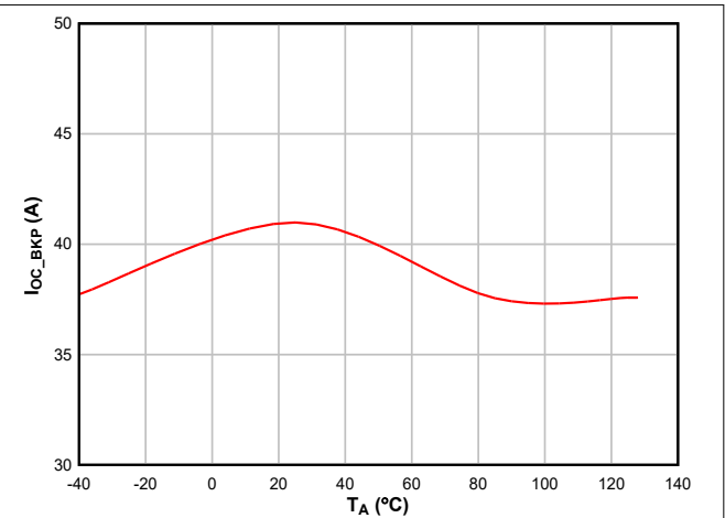
図 6-14. 温度範囲にわたるバックアップ過電流保護スレッシュホルド
