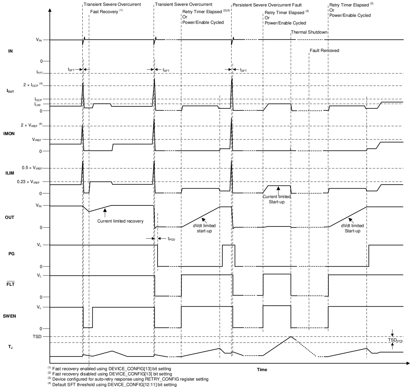
図 7-5. 短絡応答
