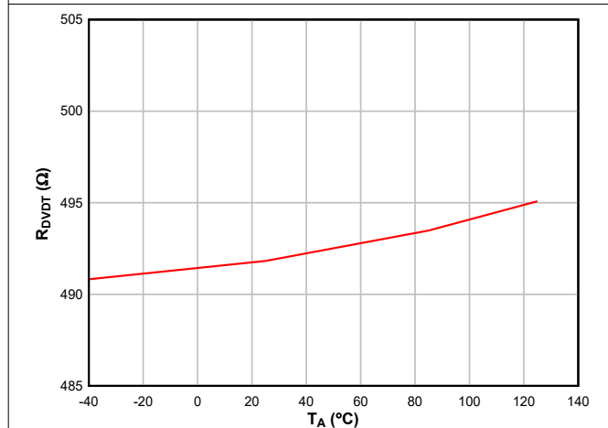
図 6-17. 温度範囲にわたる DVDT 放電抵抗
