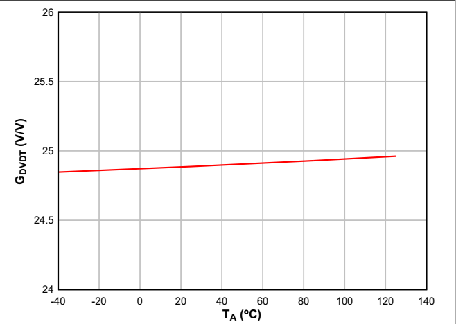
図 6-16. 温度範囲にわたる DVDT ゲイン
