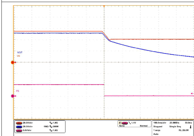
図 8-8. 低電圧保護
