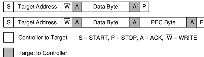
図 7-8. 送信バイト
