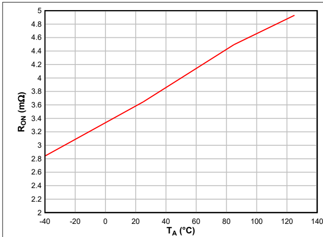
図 6-1. 温度範囲にわたる ON 抵抗
