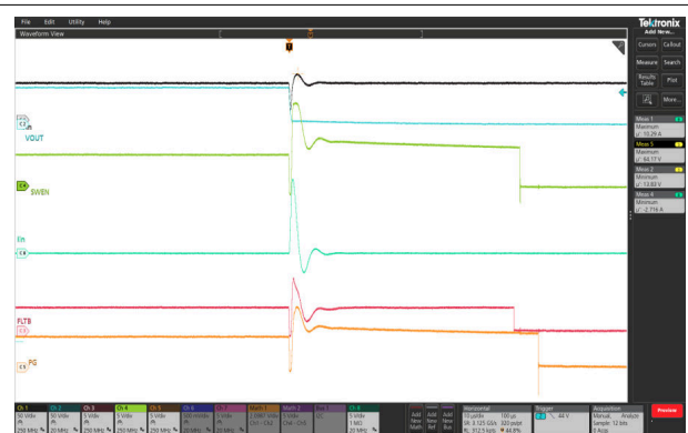
図 6-26. 過電流保護
