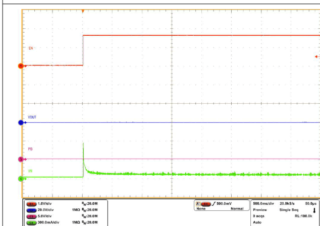
図 8-10. パワーアップ時の短絡: VIN = 54V、EN/ UVLO が 0V から 3V に昇圧
