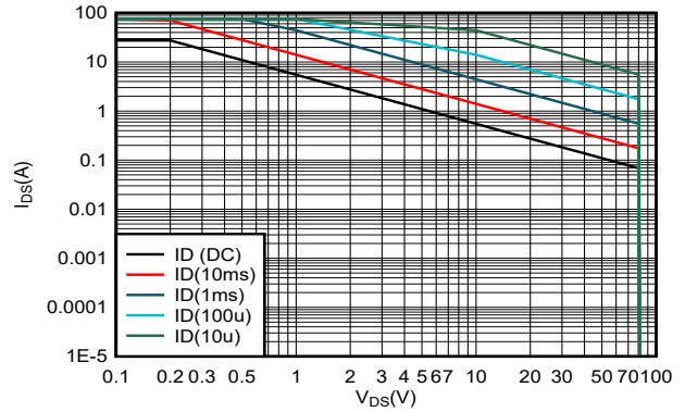
図 6-20. 定常状態の許容動作領域 (AOA)
