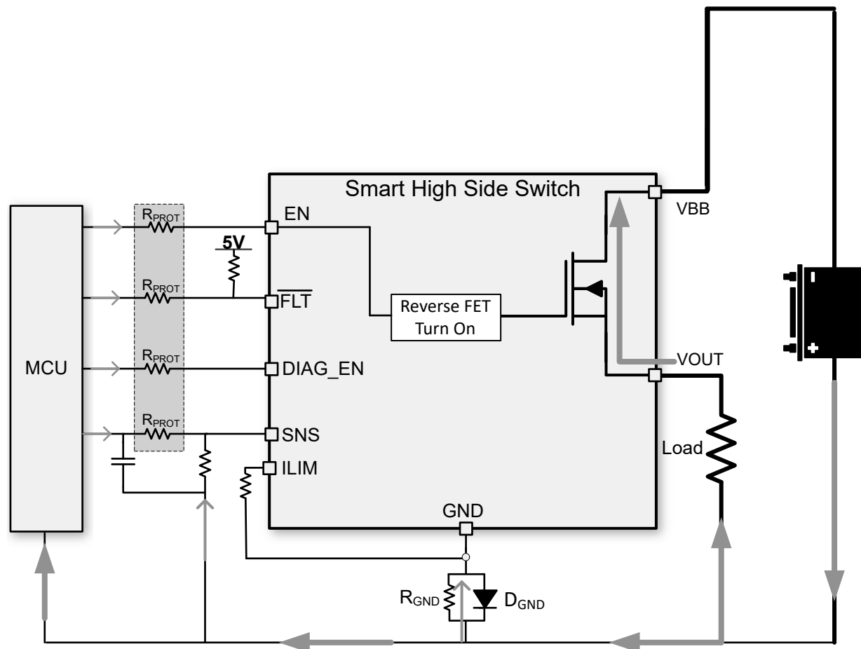
図 8-43. マイコン I/O 保護
