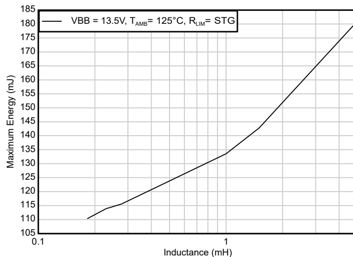
図 8-26. 誘導性スイッチオフ時の最大エネルギー吸収量とインダクタンスとの関係 (シングルパルス、VBB = 13.5V、T AMB = 125°C)
