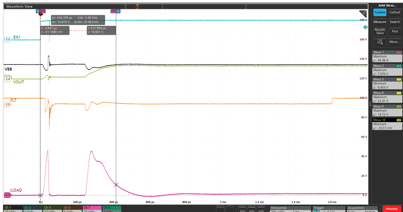
図 8-28. 13.5V の VBB、ILIM ピンを接地、周囲温度 125°C という条件における、TPS1HC04-Q1 デバイスによる 470 \mu F 容量性負荷の充電
