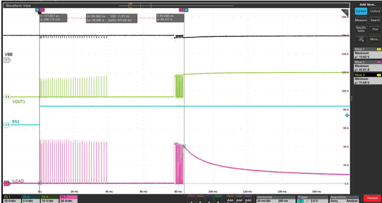
図 8-34. 13.5V VBB 条件下における TPS1HC04-Q1 シングルチャネル使用時の 100W バルブ充電特性、 T_A(\text{device}) = 25^\circ\text{C} 、 T_A(\text{bulb}) = -40^\circ\text{C} 、 ILIM = GND
