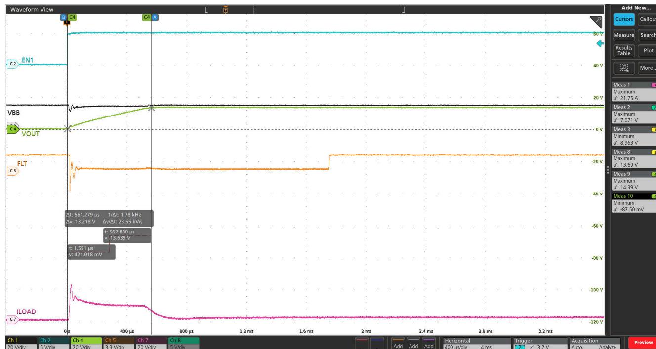
図 8-29. TPS1HC04-Q1 デバイスにおける 470µF 容量性負荷の充電 (VBB = 13.5V、ILIM ピンオープン、周囲温度 125°C)
