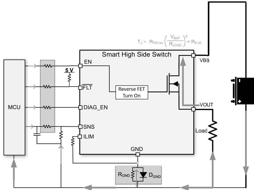
図 8-42. GND ネットワークによる逆電流保護
