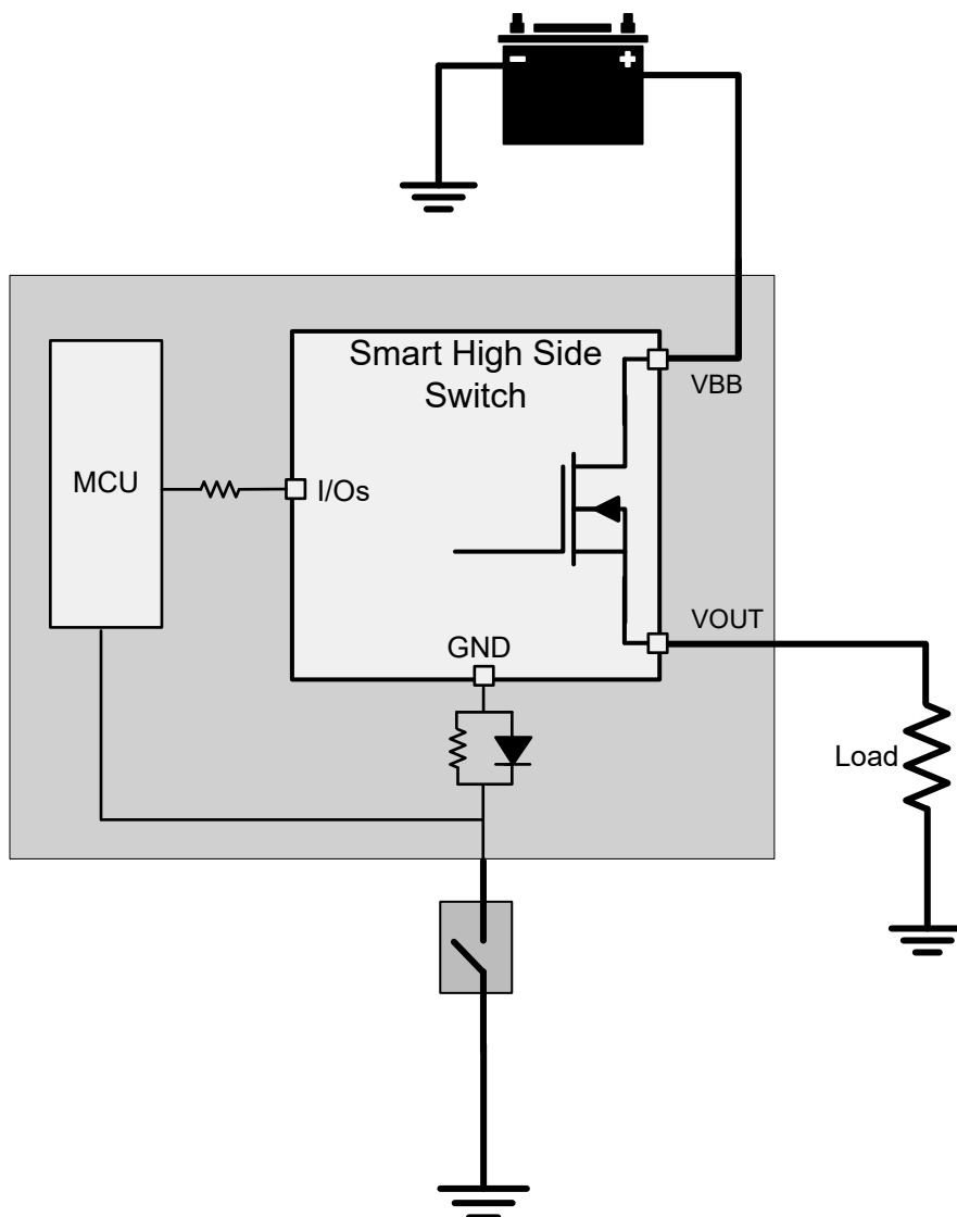
図 8-39. モジュールの GND 喪失
