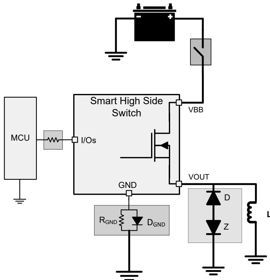
図 8-40. バッテリの損失
