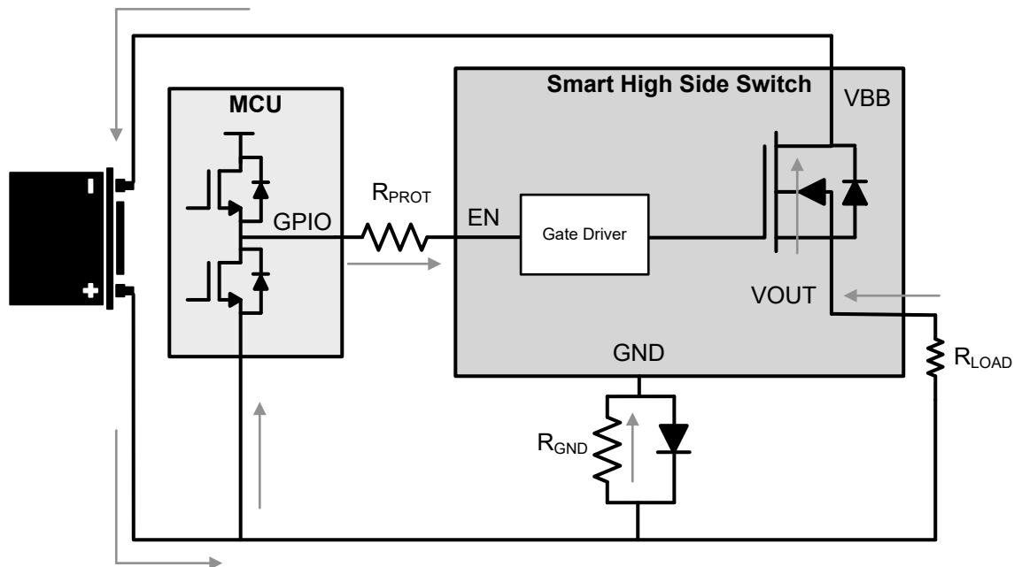
図 8-37. 逆バッテリ回路
