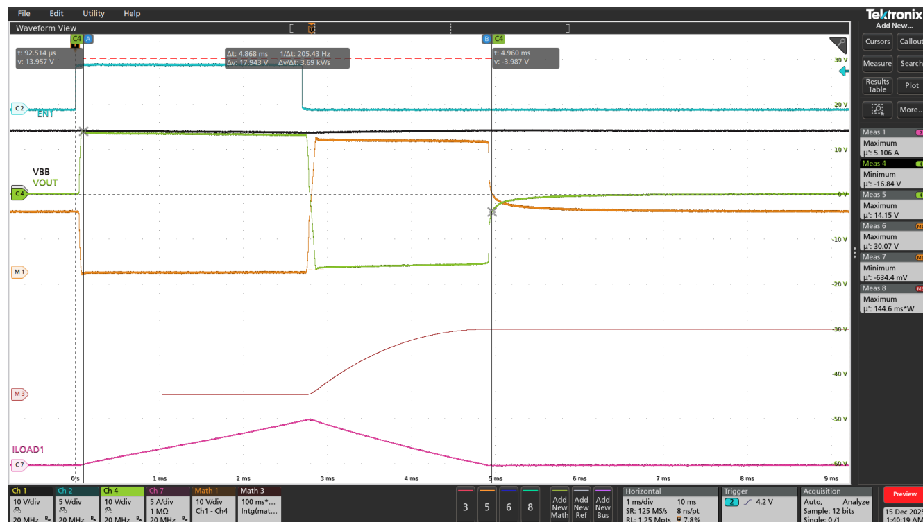
図 8-25. 5mH 誘導性負荷ドライブ (VBB = 13.5V、T AMB = 125°C)
