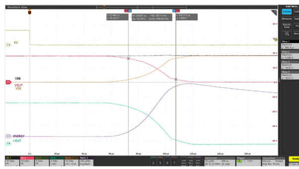
VBB = 13.5V I OUT1 = 5A T AMB = 25°C V EN = 5V ~ 0V
