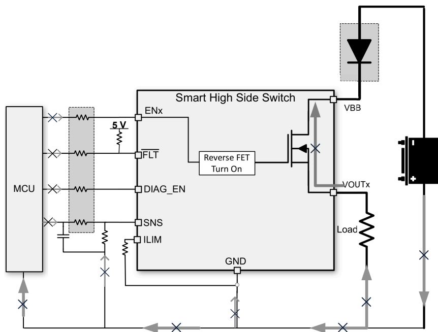
図 8-41. ブロックダイオードによる逆電流保護
