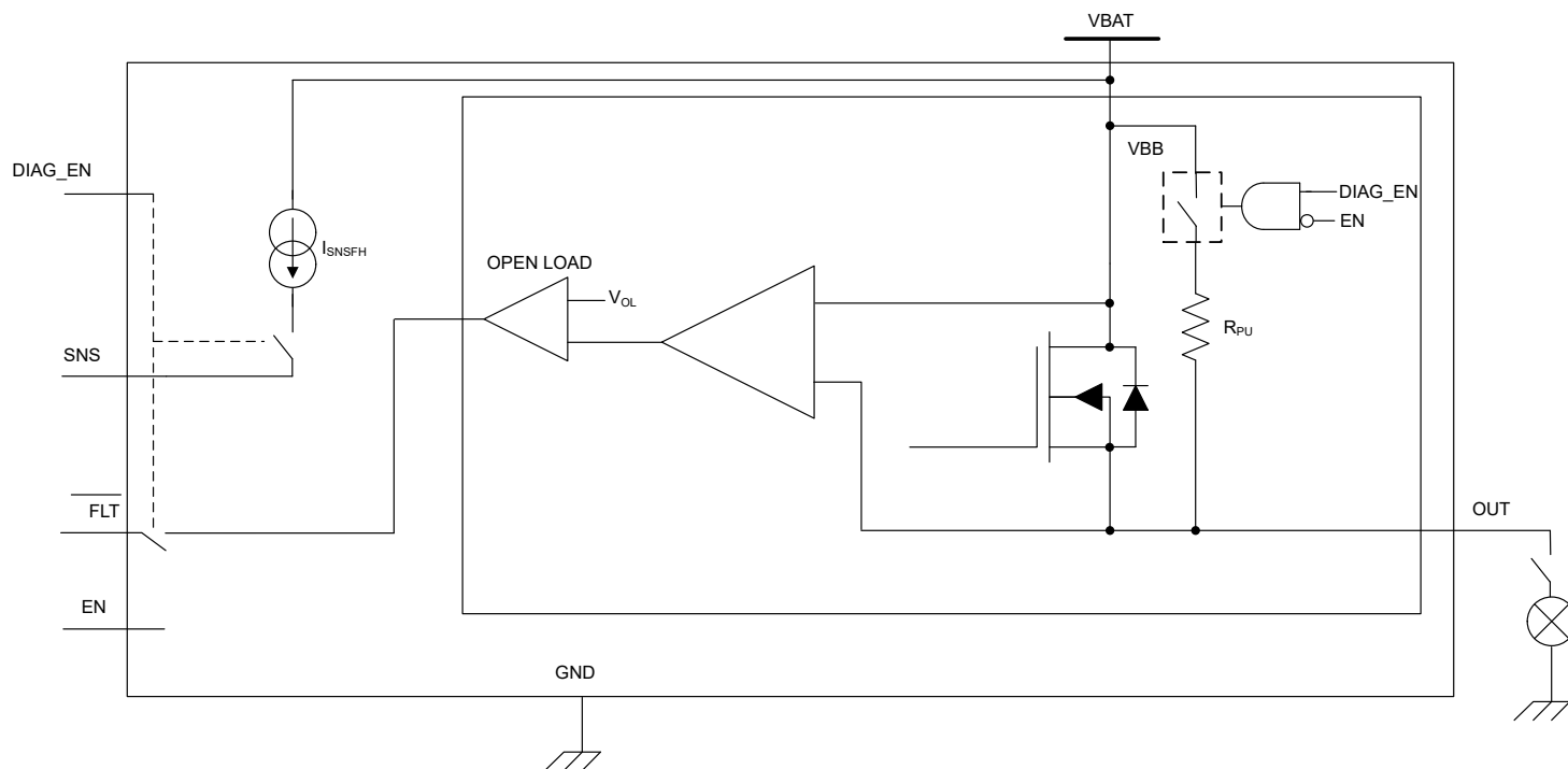
図 8-35. オフ状態での開放負荷検出
