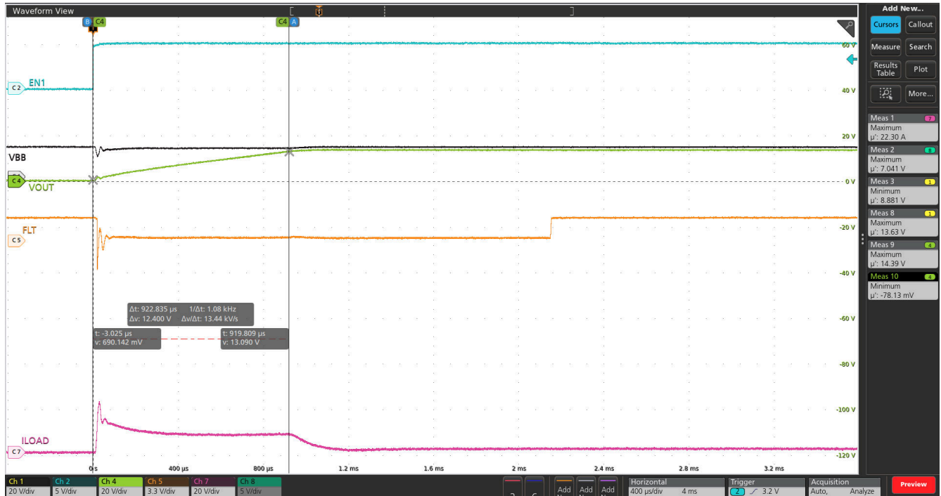
図 8-30. TPS1HC04-Q1 デバイスにおける 680µF 容量性負荷の充電 (VBB = 13.5V、ILIM ピンオープン、周囲温度 125°C)
