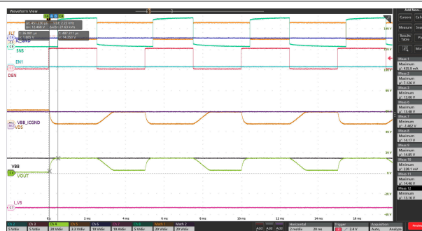
VBB = 13.5V V OUT = 開放負荷 T AMB = 25°C DIAG_EN = PWM V EN1 = 0V (200Hz)
