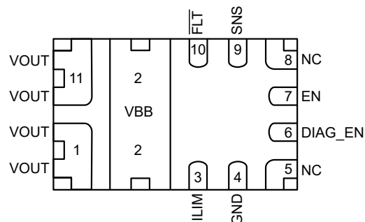
図 5-1. VAH パッケージ TPS1HC04-Q1 上面図
