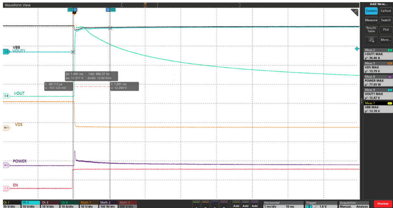
図 8-33. 13.5V VBB 条件下における TPS1HC04-Q1 シングルチャネル使用時の 35W パルプ充電特性、 T_A (device) = 25°C、 T_A (bulb) = -40°C、ILIM = GND
