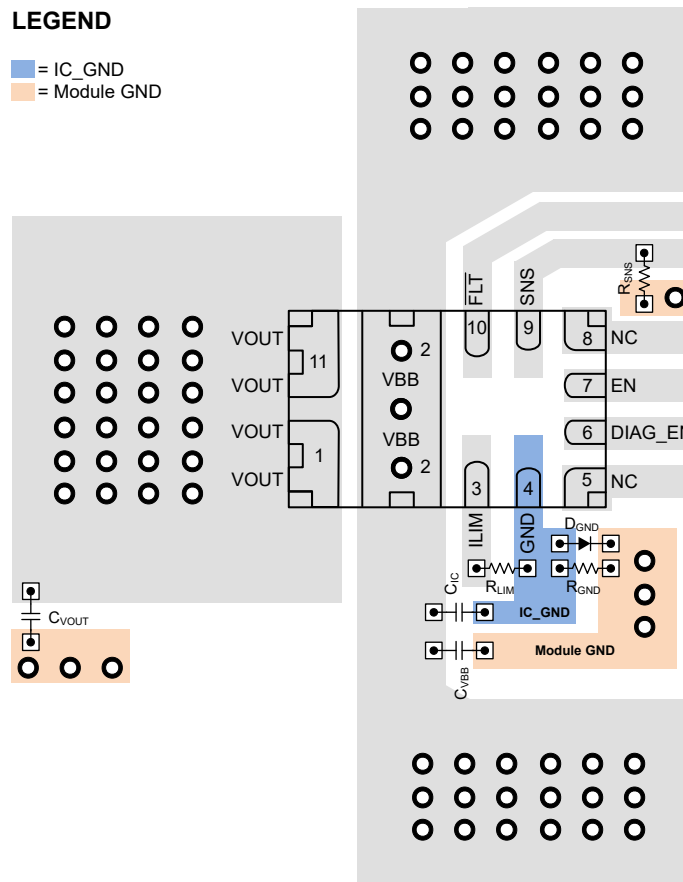
図 9-14. GND ネットワークを使ったレイアウト例
