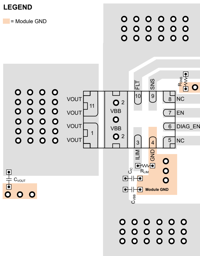
図 9-13. GND ネットワークを使わないレイアウト例
