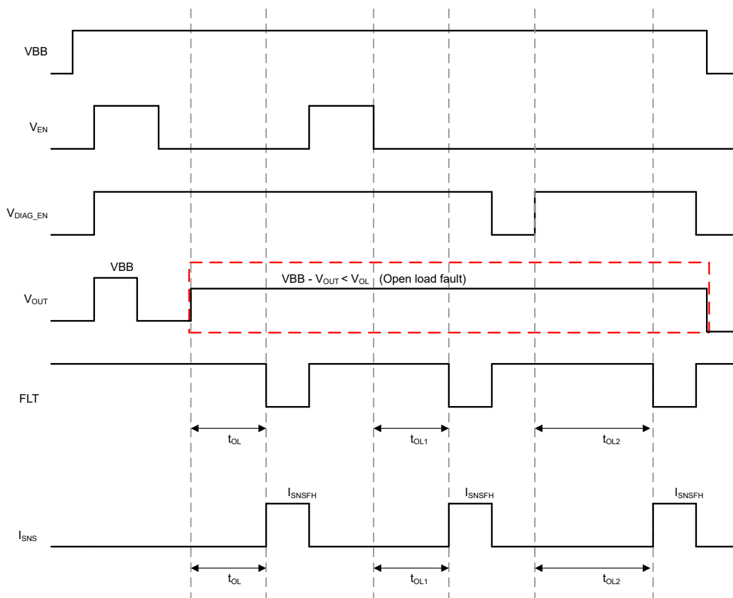
図 8-35. オフ状態での開放負荷検出
