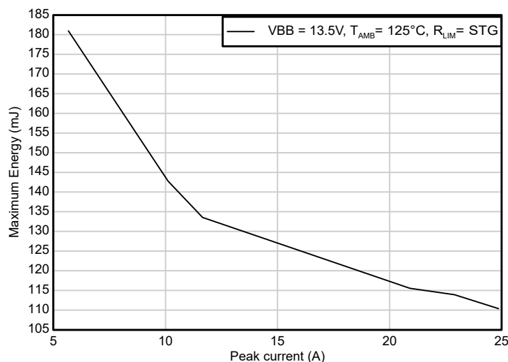
図 8-27. 誘導性スイッチオフ時の最大エネルギー吸収量とピーク電流との関係 (シングルパルス、VBB = 13.5V、T AMB = 125°C)
