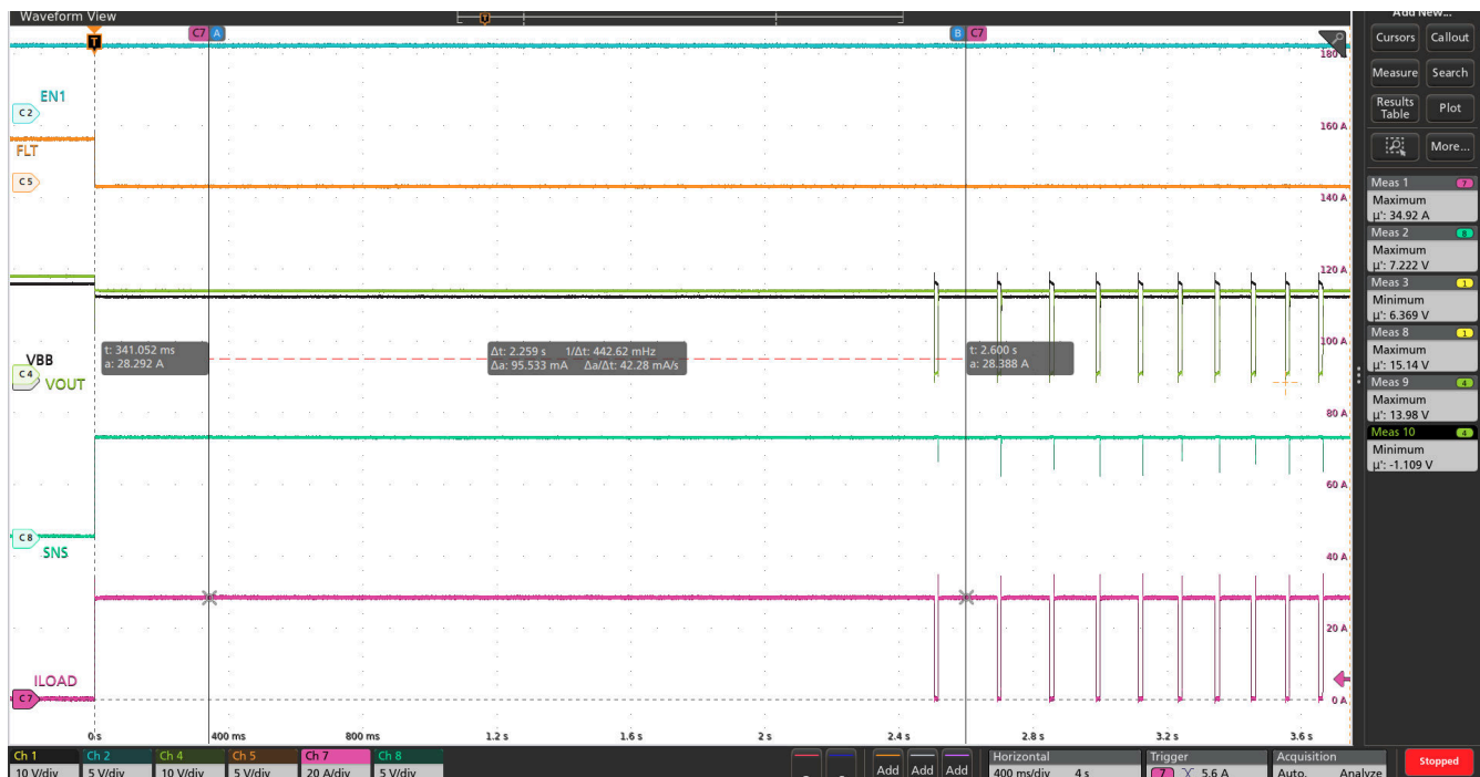
図 8-18. デバイスは電流制限 ( I_{\text{LIM}}=\text{GND} ) 未満の負荷電流 (28A 電子負荷) における無限サーマルシャットダウンの再試行動作を開始します
