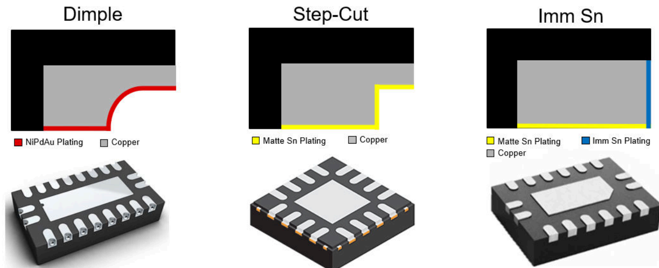
図 9-15. ウェットブル フランク パッケージの種類
