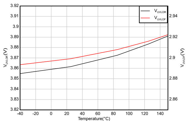
図 6-22. 低電圧誤動作防止スレッショルド ( V_{UVLOR} 、 V_{UVLOF} ) と温度との関係
