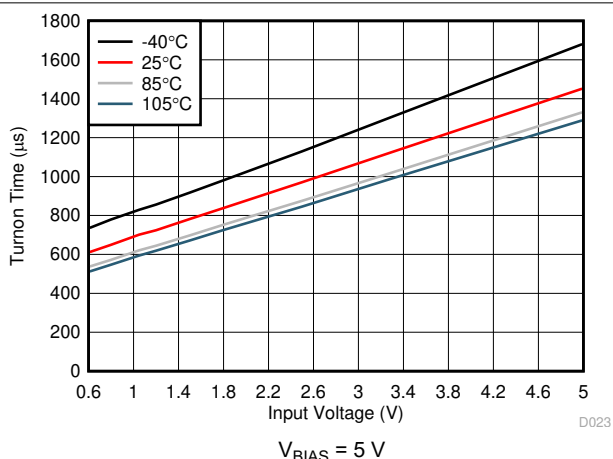
6-28. Turnon Time vs Input Voltage
