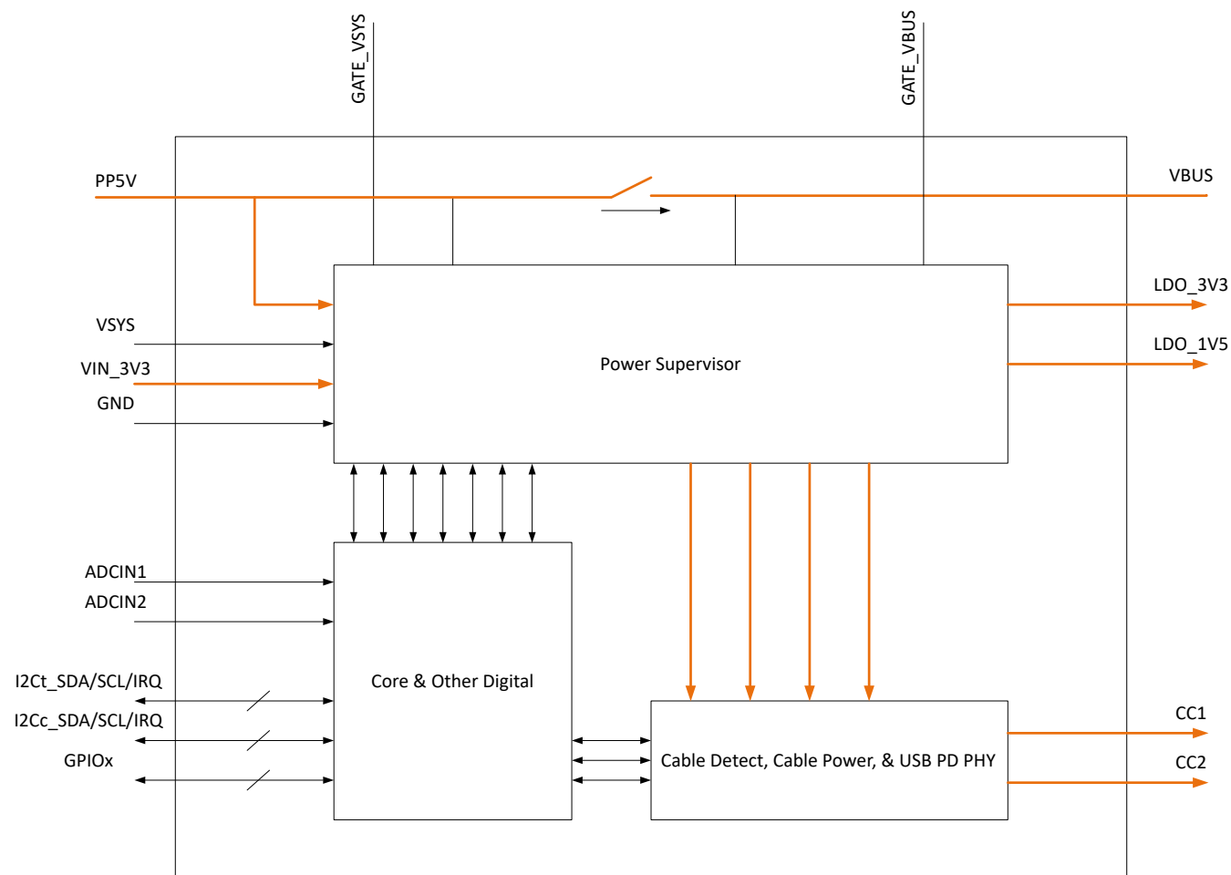
図 8-2. TPS25751S
