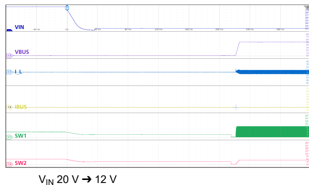
図 9-28. V_{IN(OVP)} Recovery
