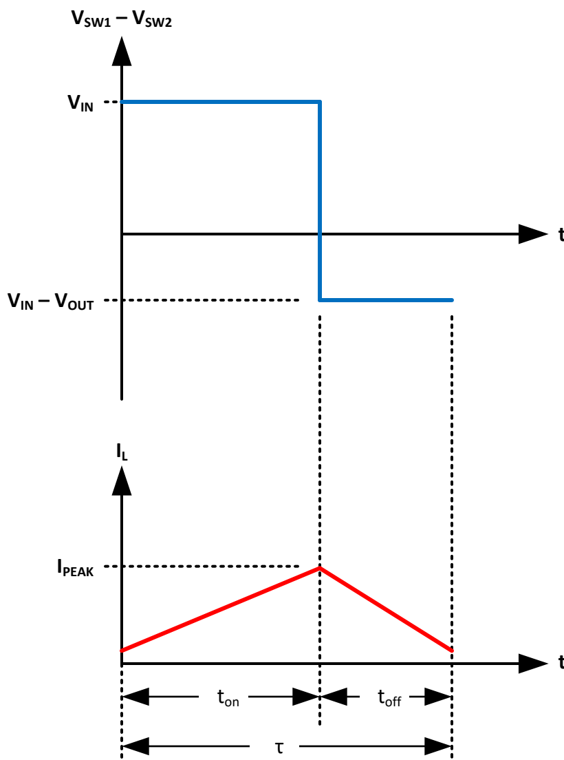
図 8-12. Boost State
