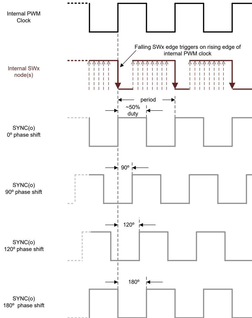
図 8-15. SYNC(o) Phase Shift
