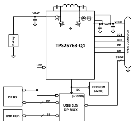
TPS25763-Q1 の概略回路図
