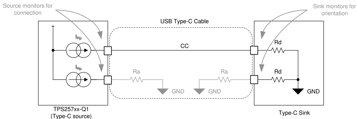
图 8-29. Type-C Cable
