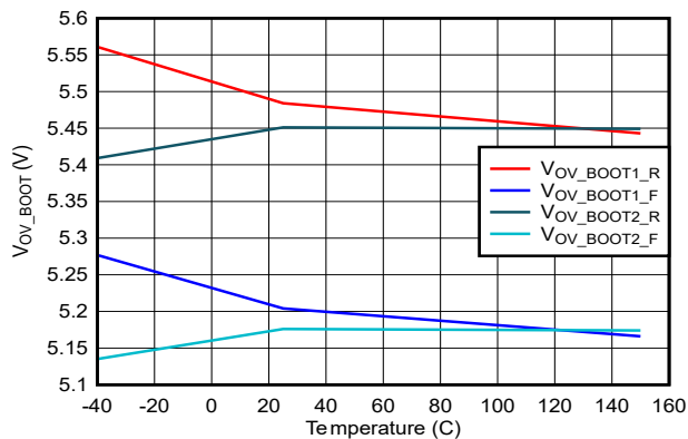
図 6-23. BOOTx OVP vs Temperature
