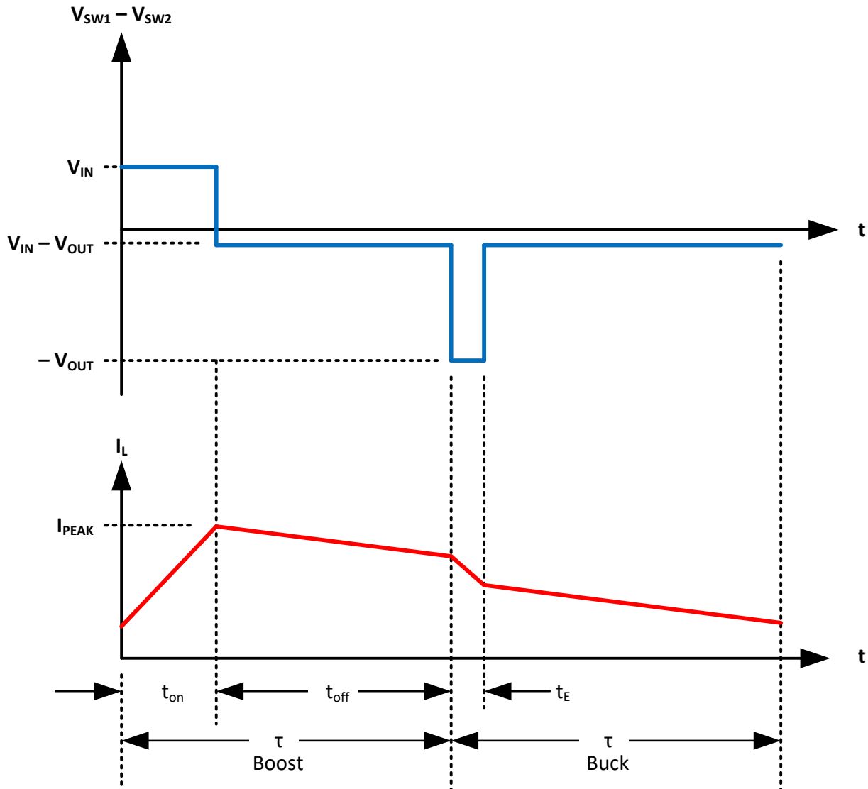
図 8-11. Boost Transition
