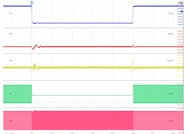
図 9-33. Load Transient (Boost): V_{BUS} = 20\text{ V}
