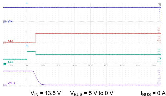
9-13. Type-C Detach
