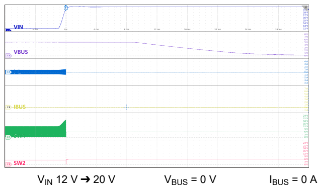
図 9-29. V_{IN(OVP)} Showing V_{BUS} Discharge
