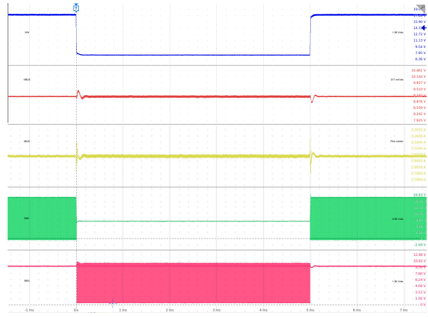
図 9-35. Line Transient: V_{BUS} = 20\text{ V}
