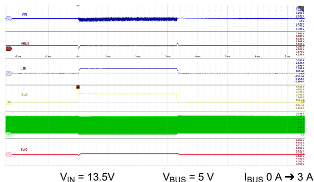
図 9-30. Load Transient (Buck): V_{BUS} = 5\text{ V}
