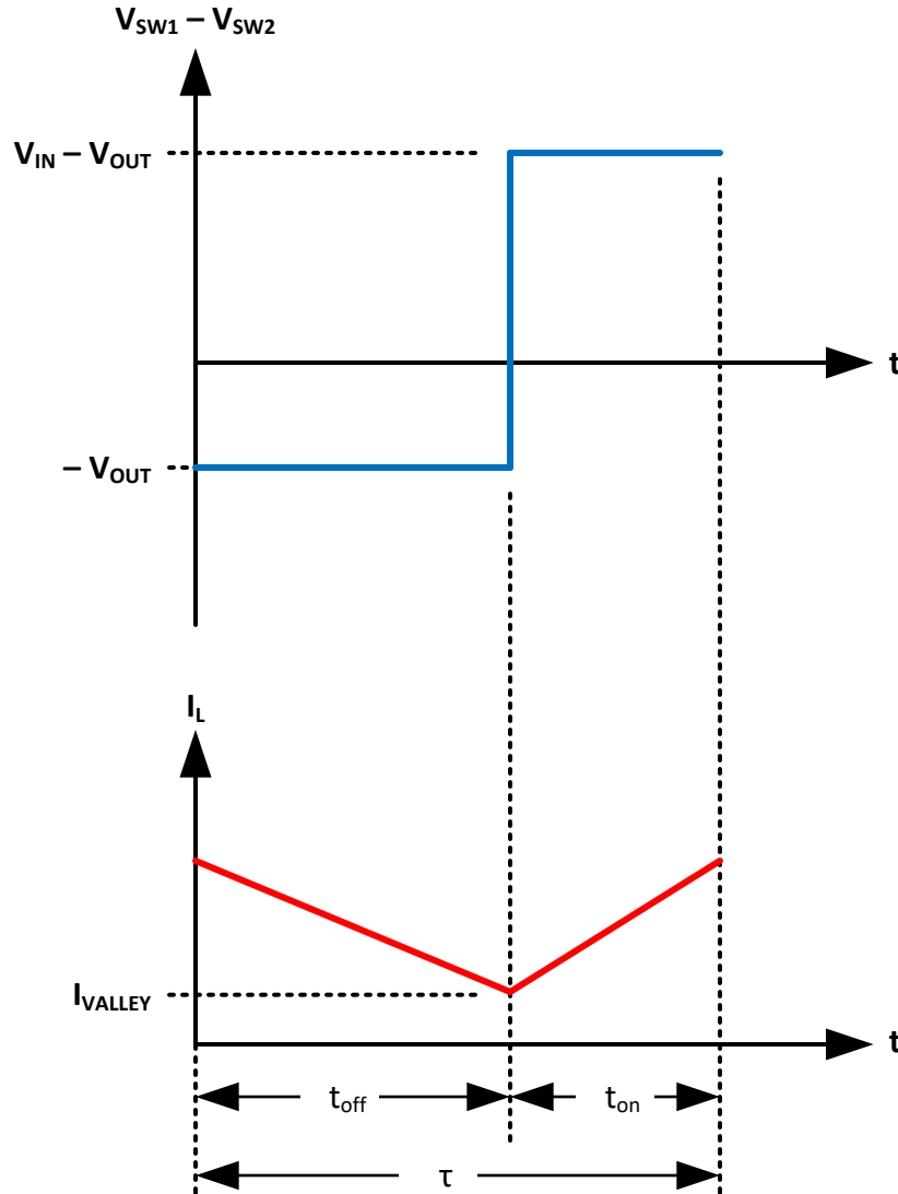
図 8-9. Buck State
