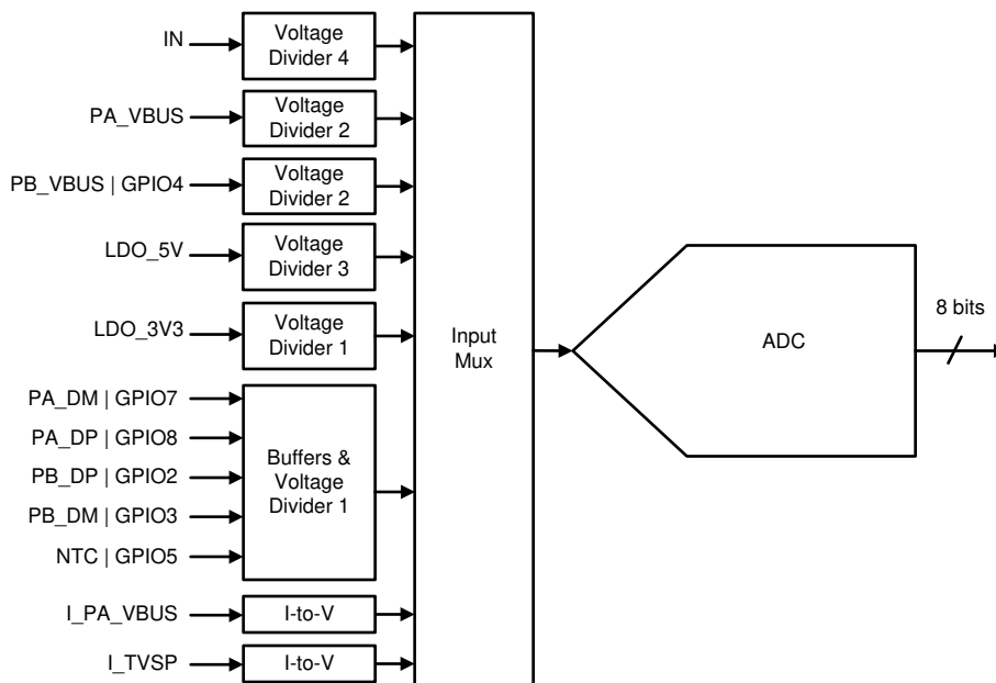
図 8-31. SAR ADC
