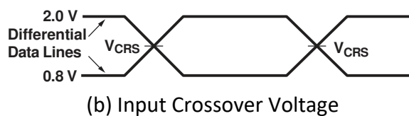
図 7-4. USB Endpoint Crossover Voltages
