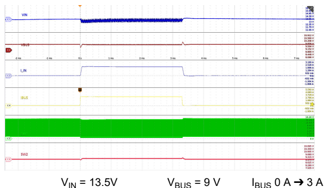
図 9-31. Load Transient (Buck): V_{BUS} = 9\text{ V}
