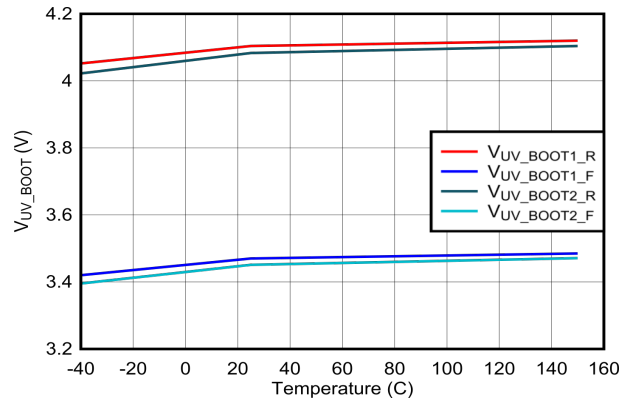
図 6-22. BOOTx UVLO vs Temperature
