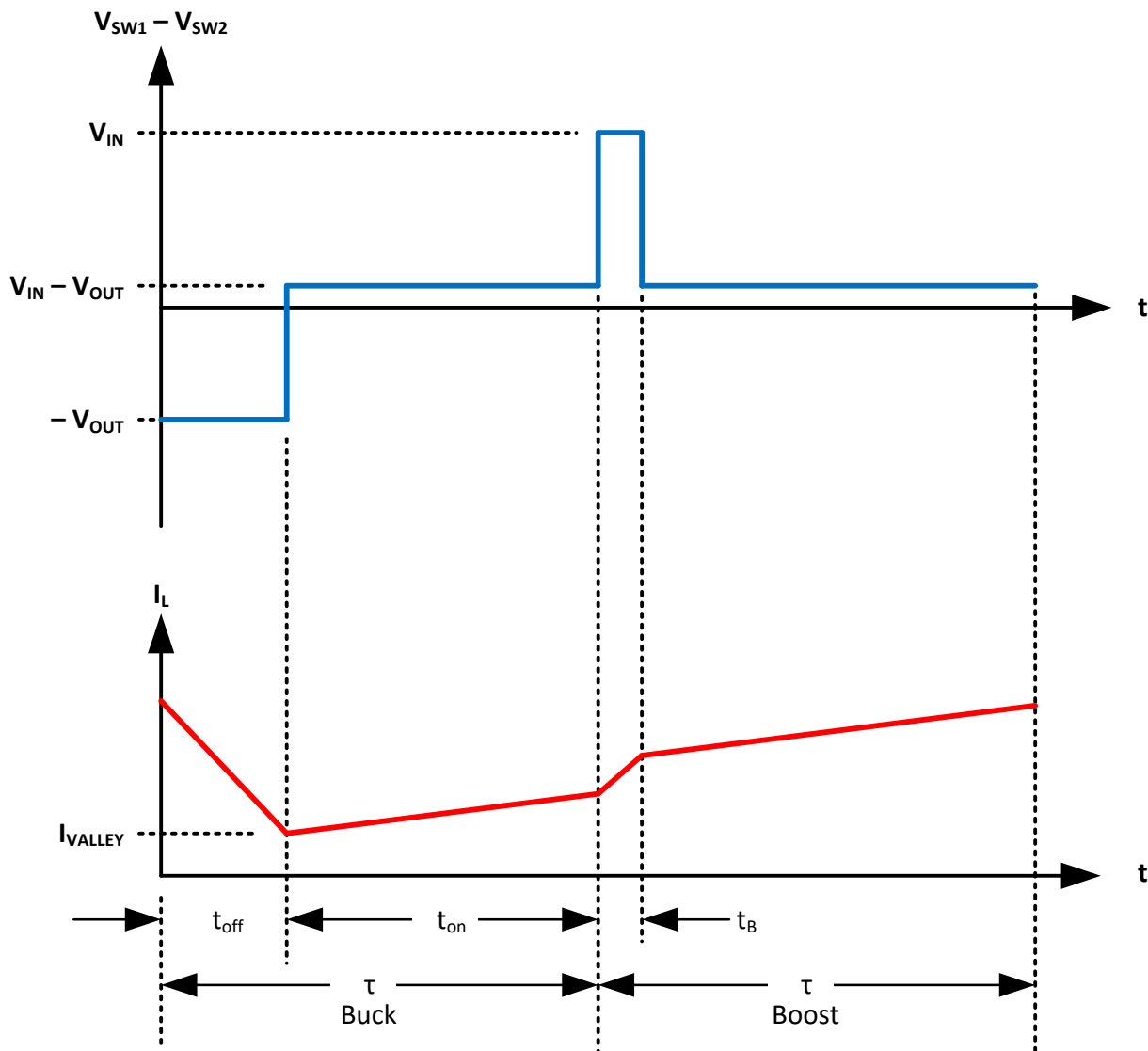
図 8-10. Buck Transition
