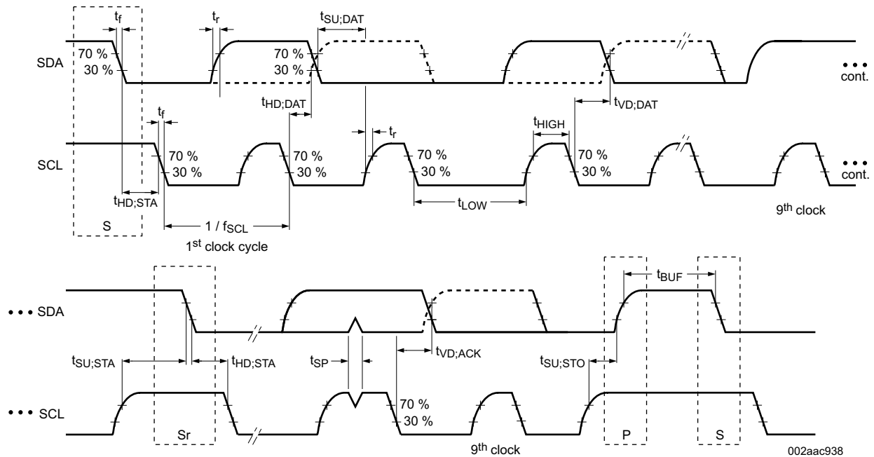
図 7-1. I²C Target Interface Timing
