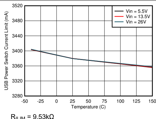
図 8-12. 接合部温度に対する USB 電源スイッチ電流制限
