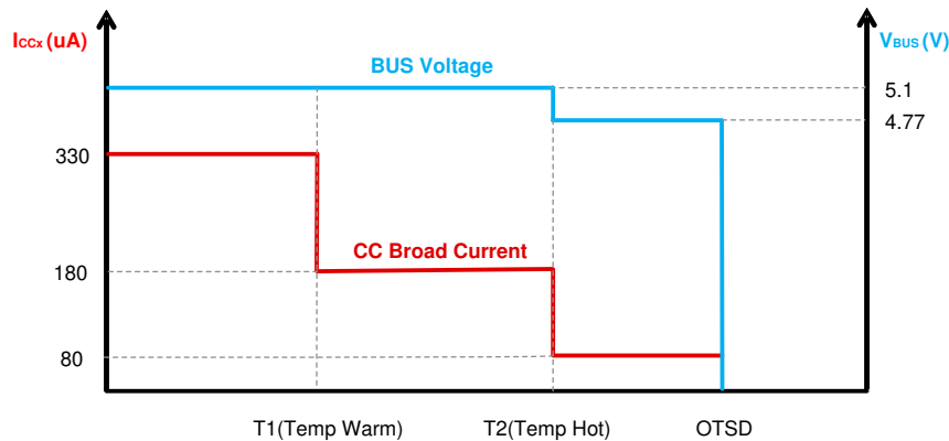
図 10-11. 温度ウォームと温度ホット・スレッショルドが発生したときの TPS25858-Q1 の動作
