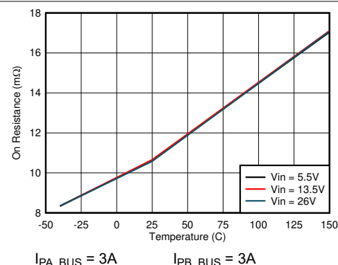
図 8-10. 接合部温度に対する上限側 MOSFET オン抵抗
