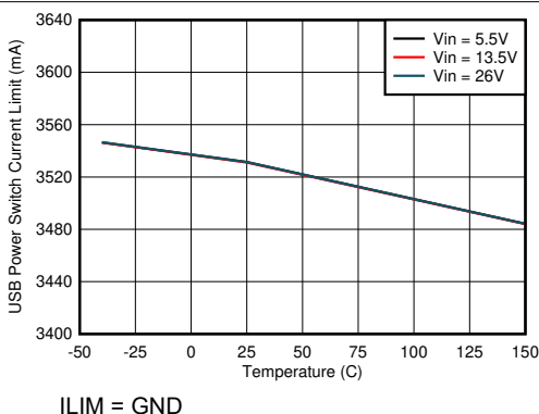
図 8-11. 接合部温度に対する USB 電源スイッチ電流制限
