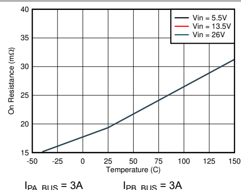
図 8-9. 接合部温度に対する下限側 MOSFET オン抵抗
