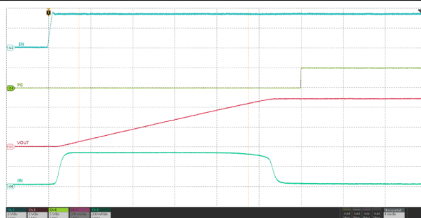
図 6-32. Input Hot-Plug
