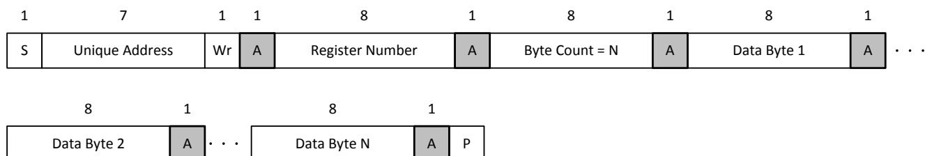
図 8-32. I 2 C 固有アドレス書き込みレジスタ プロトコル
