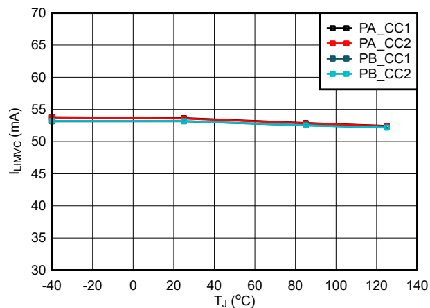
図 6-8. VCONN スイッチの電流制限。
