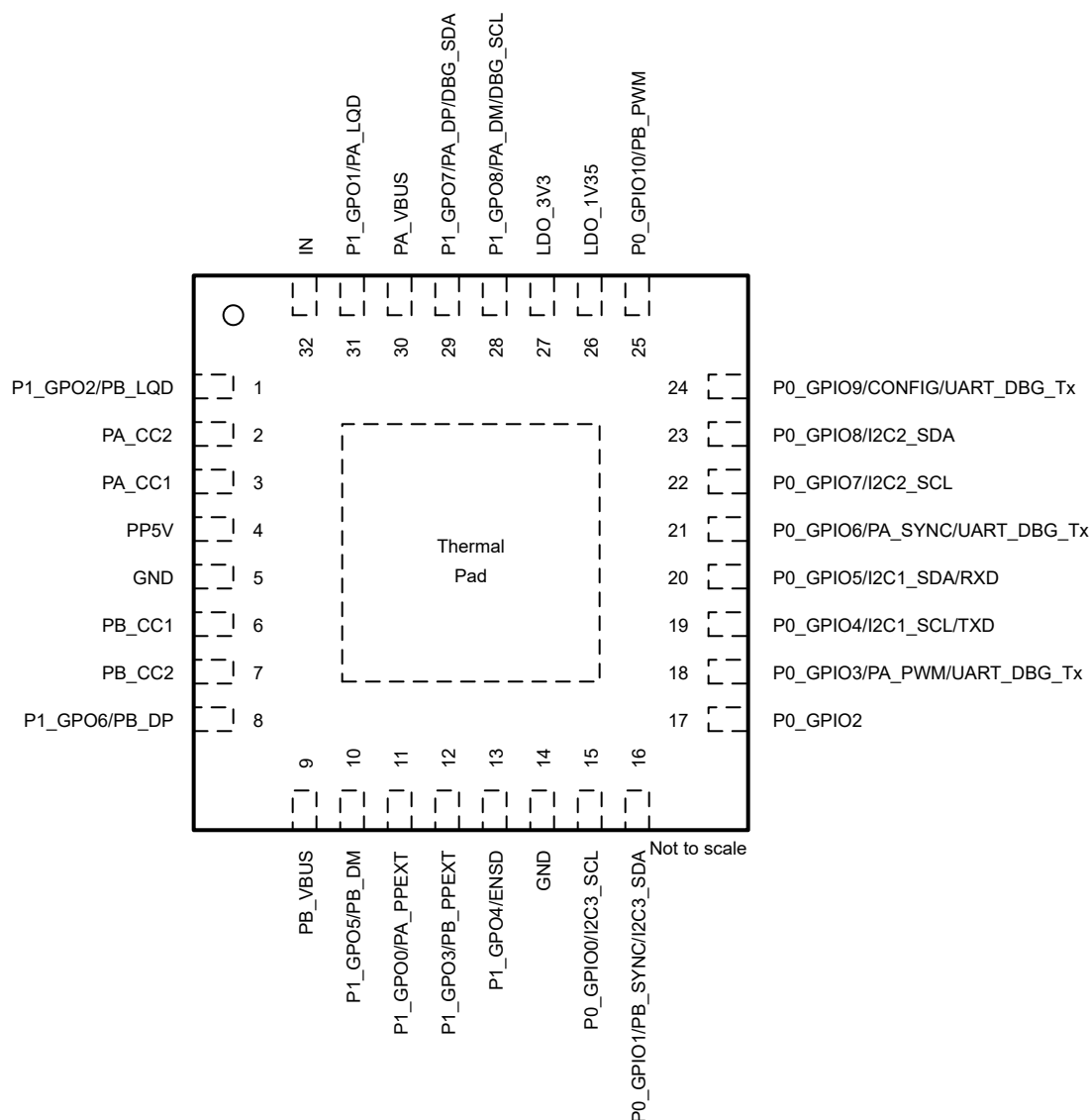
図 5-1. TPS26742-Q1 RHB パッケージ、32 ピン QFN (上面図)
