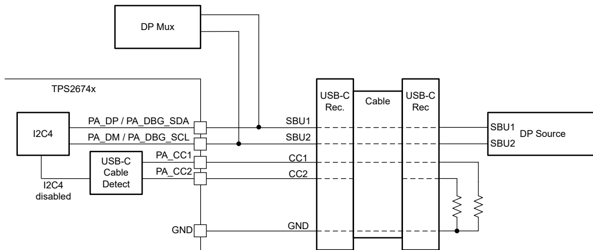
図 8-18. I2C4 は SBU 信号に干渉
