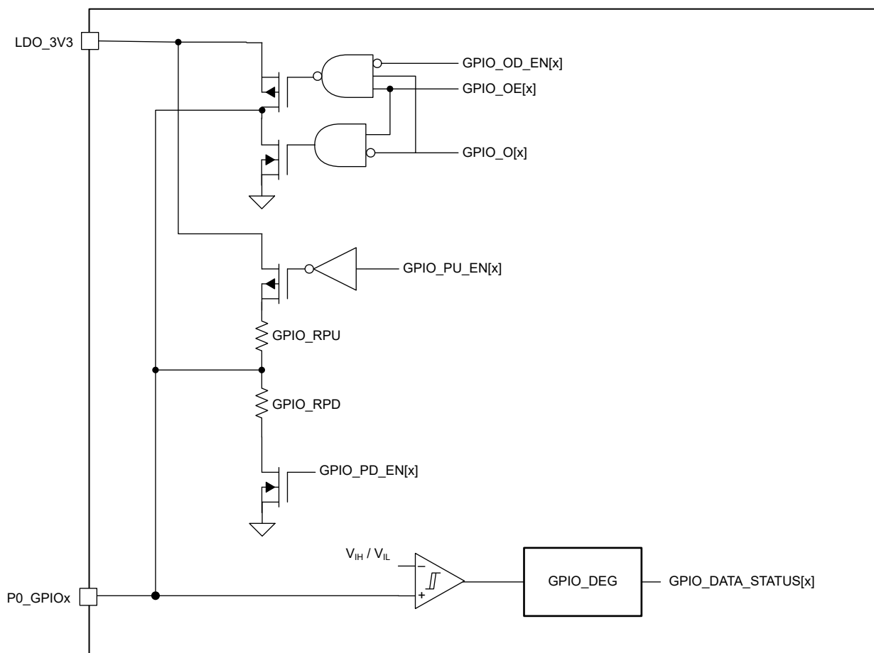
図 8-25. P0_GPIOx バッファの図
