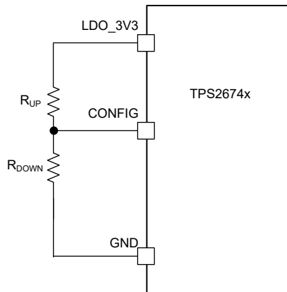
図 8-36. I2C_ADDR ピンの構成
