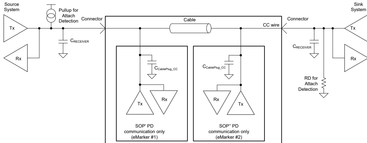
図 8-13. USB-PD マルチドロップ構成の例
