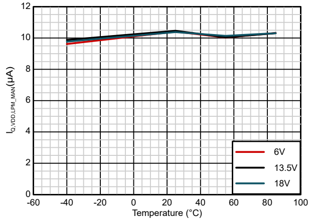
MANUAL_LPM 状態 VDD = 5V チャンネル オフ IOUT = 0A
