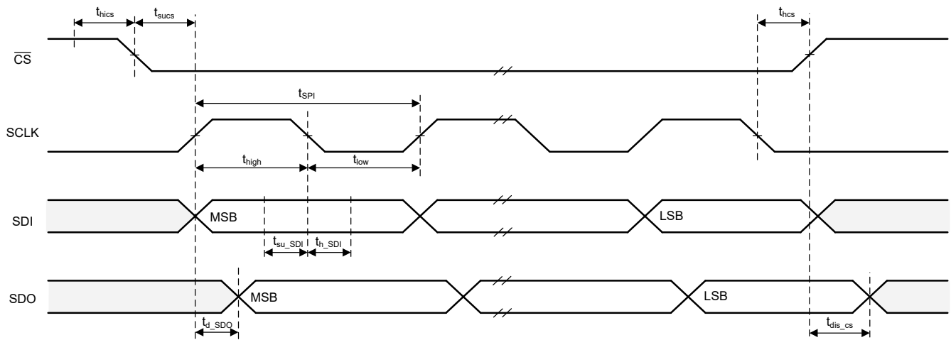
図 7-2. SPI のタイミング特性の定義
