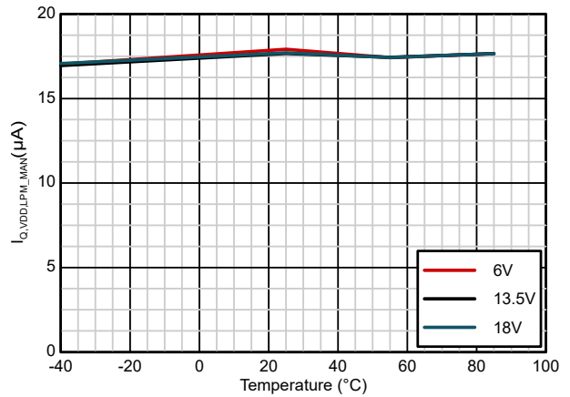
MANUAL_LPM 状態 VDD = 5V 両方のチャンネルがイネーブル IOUT = 0A
