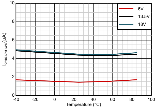
MANUAL_LPM 状態 VDD = 5V チャンネル オフ
