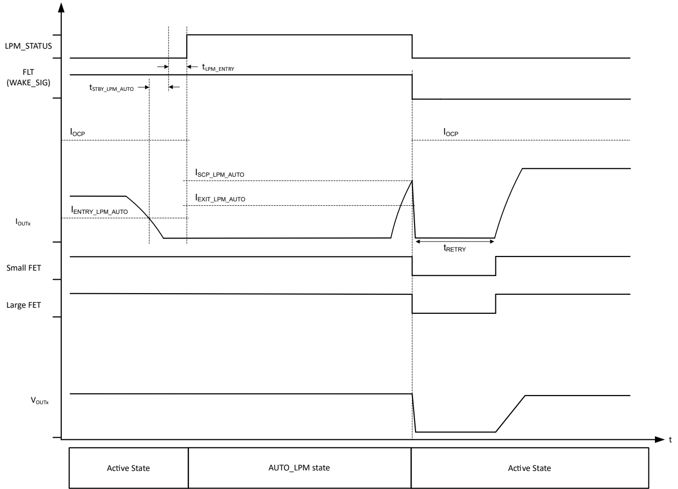
図 8-35. AUTO_LPM 状態で、 I_{SCP\_LPM\_AUTO} を超え、 I_{OCP} 未満の負荷増加
