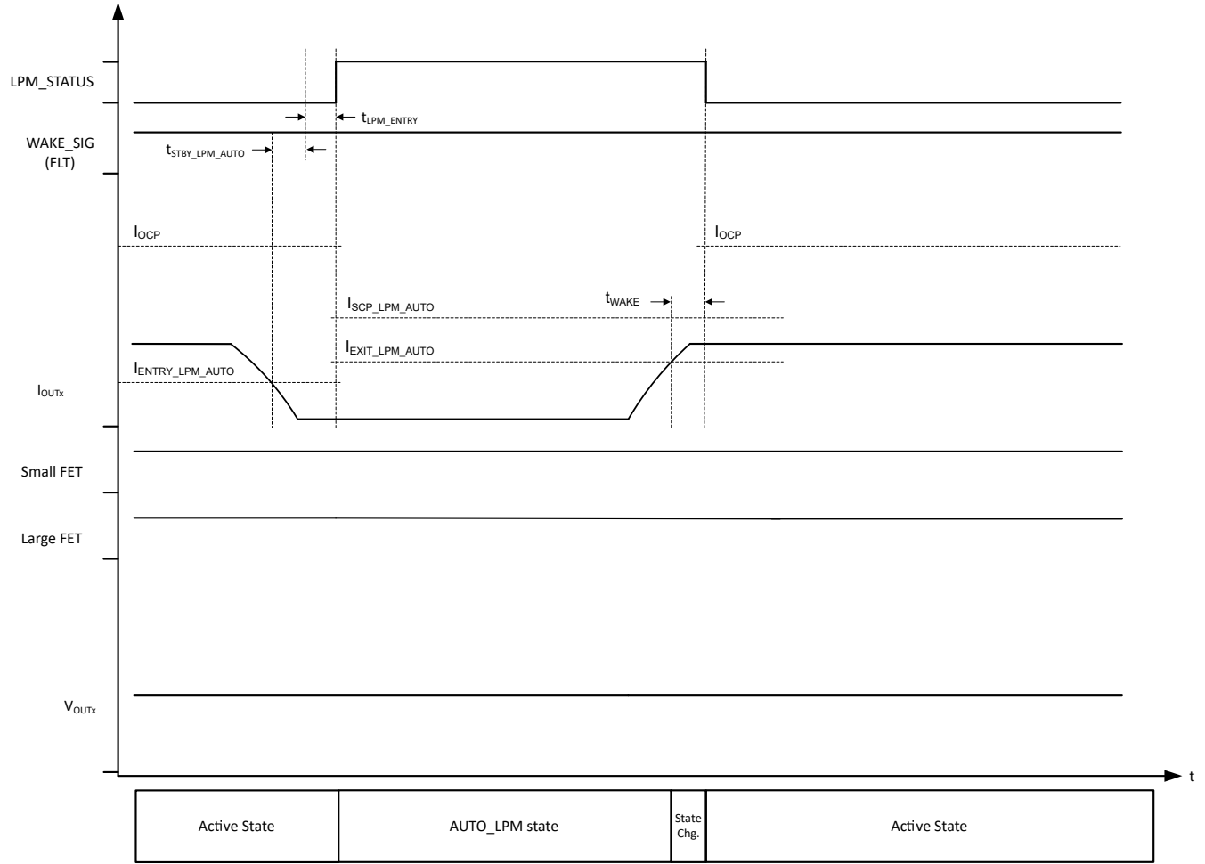
図 8-34. AUTO_LPM 状態で、 I_{EXIT\_LPM\_AUTO} を超え、 I_{SCP\_LPM\_AUTO} 未満の負荷増加
