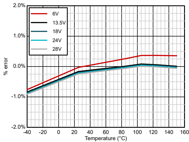
k_{SNS1} リファレンス = 5000 OL_ON_EN_CHx = 0 IOUT = 2A
