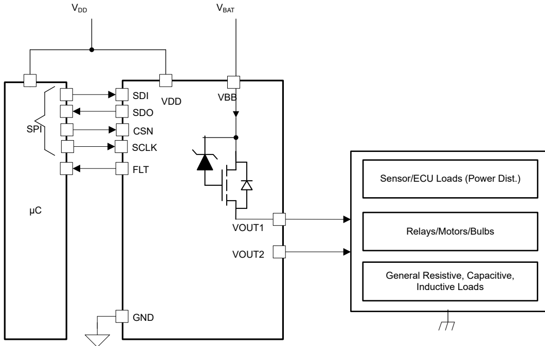
概略回路図
