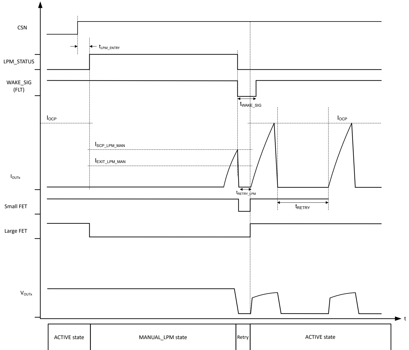
図 8-33. MANUAL_LPM 状態で、I OCP を上回る負荷増加
