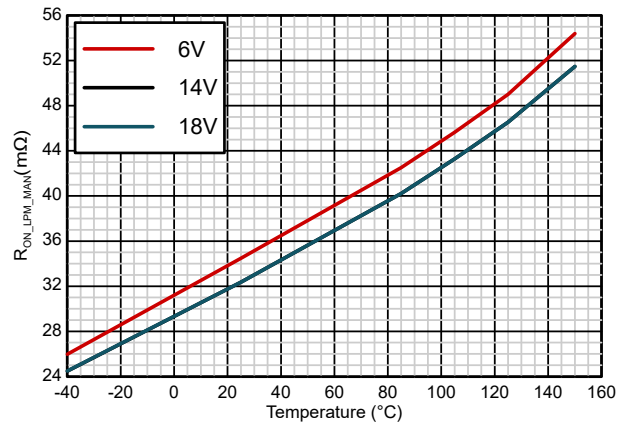
図 6-4. MANUAL_LPM のオン抵抗 ( R_{ON\_LPM\_MAN} ) と温度との関係
