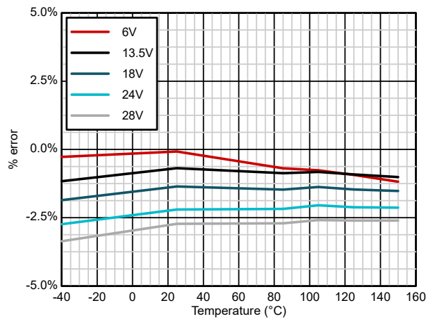
k_{SNS2} リファレンス = 1400 OL_ON_EN_CHx = 1 IOUT = 25mA
