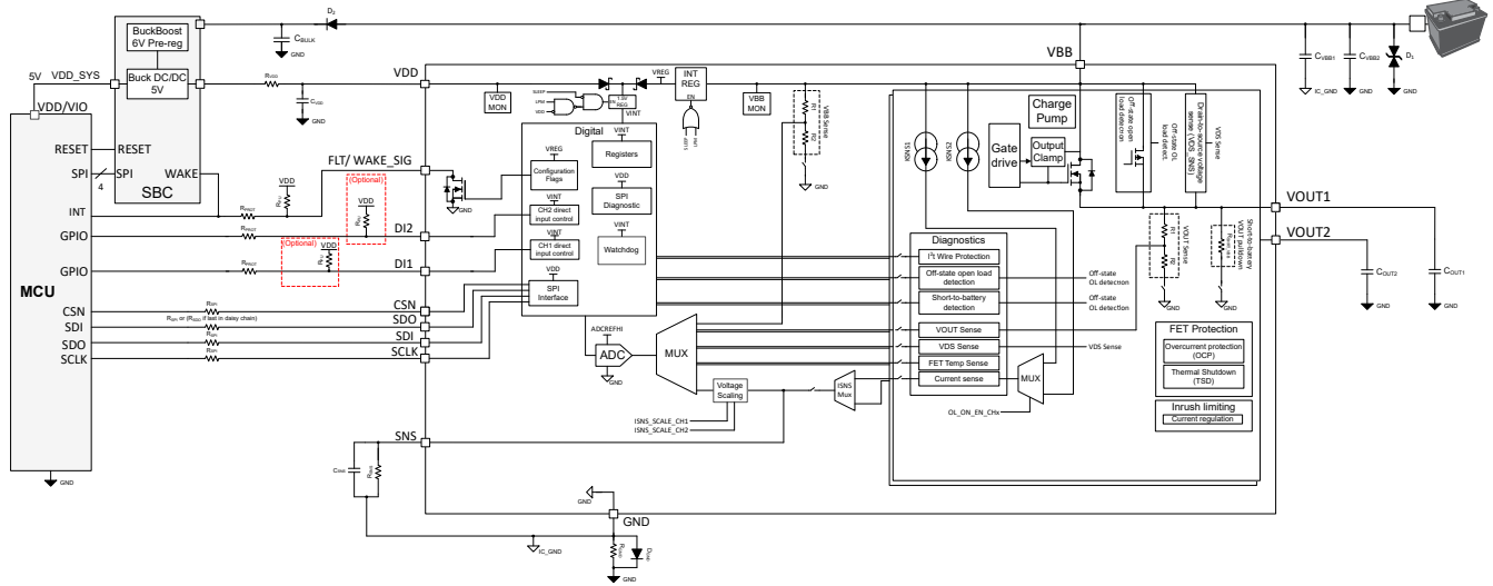
図 9-2. システム図 - TPS2HCS10B-Q1
