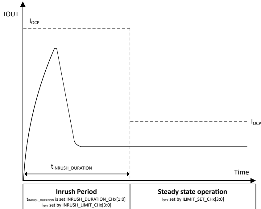
図 8-5. 容量性充電なし (CAP_CHRG_CHx [1:0] = 00) - 電球駆動例
