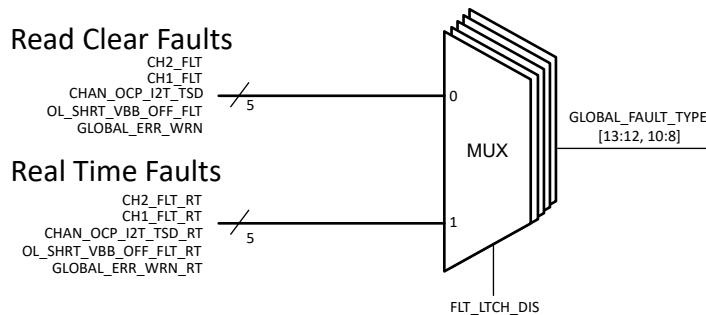
図 8-29. FLT_LTCH_DIS の実装
