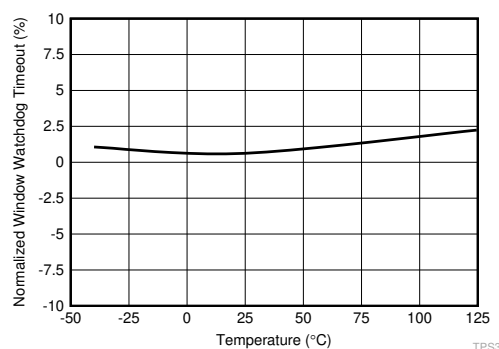
正規化されたウォッチドッグ・タイムアウト ( t_{WD} ) 精度 (SET1 = 1、CWD = NC)
