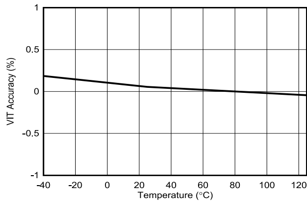
図 6-5. 変動 V_{IT} の精度と温度との関係
