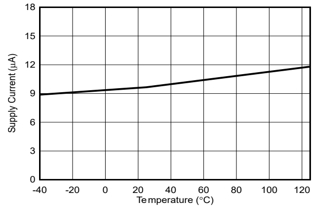
図 6-4. AOUT が有効の状態での I_{DD} と温度との代表的な関係 ( V_{DD} = 48\text{V} )
