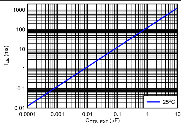
图 7-5. T_{CTS} vs C_{CTS}
