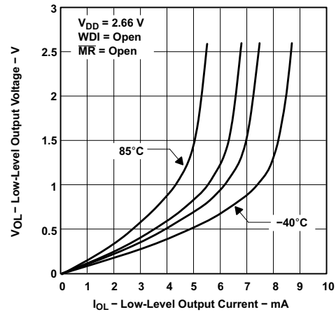
図 6-5. LOW レベル出力電圧と LOW レベル出力電流との関係
