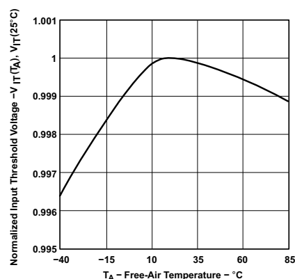
正規化された入カスレッシュホルド電圧と自由通気温度との関係
