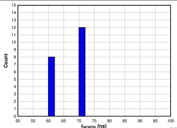
図 6-24. -40°Cでの TPS3823A-33 デバイスの WDI パルス幅ヒストグラム (ユニット数 = 20)
