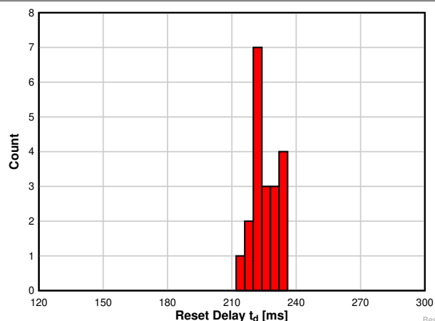
図 6-11. 125°Cでの TPS3823A-33 デバイスのリセット遅延ヒストグラム (ユニット数 = 20)
