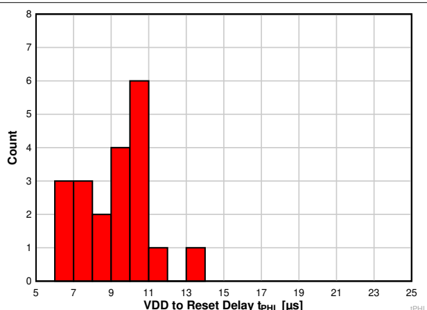
図 6-17. 125°Cでの TPS3823A-33 デバイスの VDD からリセットまでの遅延ヒストグラム (ユニット数 = 20)
