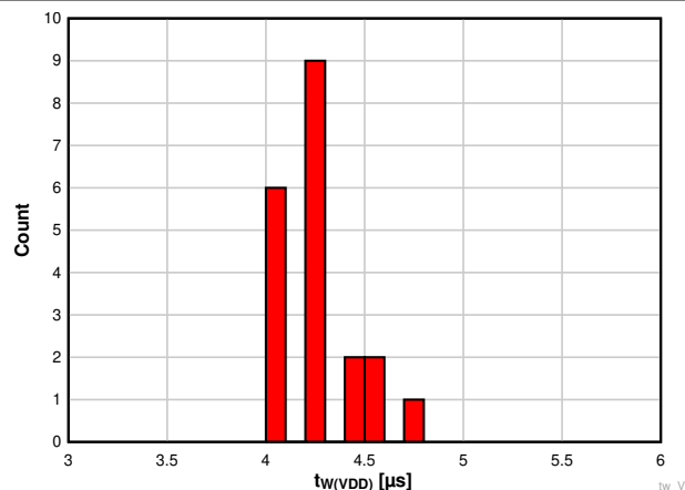
図 6-20. 125°Cでの TPS3823A-33 デバイスの VDD パルス幅ヒストグラム (ユニット数 = 20)
