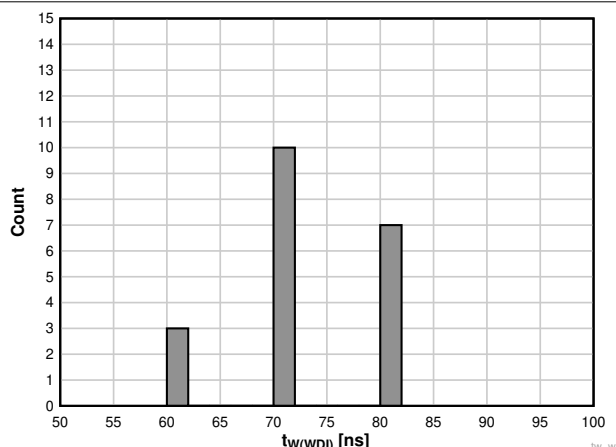
図 6-25. 25°Cでの TPS3823A-33 デバイスの WDI パルス幅ヒストグラム (ユニット数 = 20)
