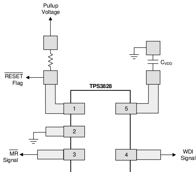
図 8-5. レイアウト例 (DBV パッケージ)
