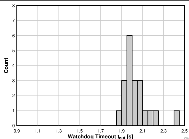
図 6-13. 25°Cでの TPS3823A-33 デバイスのウォッチドッグ・タイムアウト・ヒストグラム (ユニット数 = 20)
