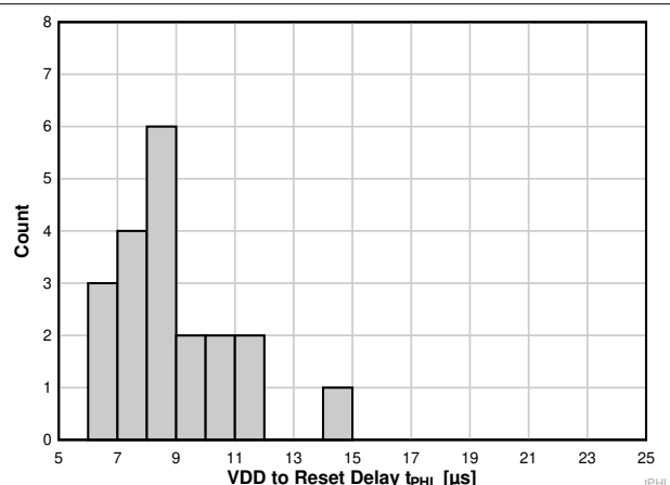
図 6-16. 25°Cでの TPS3823A-33 デバイスの VDD からリセットまでの遅延ヒストグラム (ユニット数 = 20)
