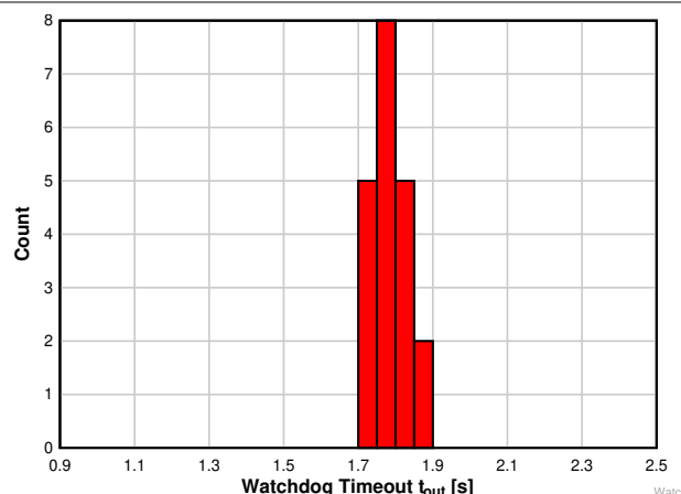
図 6-14. 125°Cでの TPS3823A-33 デバイスのウォッチドッグ・タイムアウト・ヒストグラム (ユニット数 = 20)
