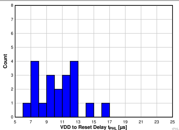
図 6-15. -40°Cでの TPS3823A-33 デバイスの VDD からリセットまでの遅延ヒストグラム (ユニット数 = 20)
