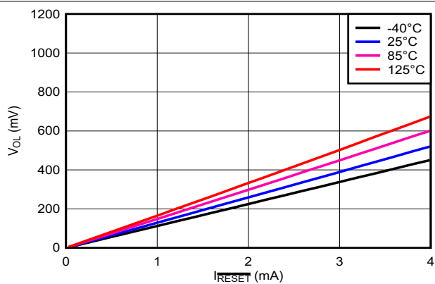
図 6-9. RESET 電流 (シンク) と V_{OL} ( V_{DD} = 12\text{V} ) との関係
