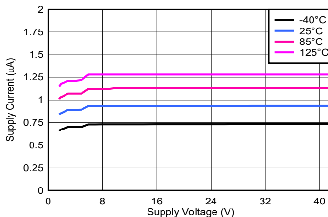
電源電圧と電源電流との関係
