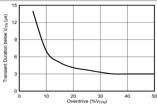
図 6-7. センス時の過渡持続時間とセンス閾値オーバードライブ電圧との関係 ( \text{CTS} = \text{Open} )
