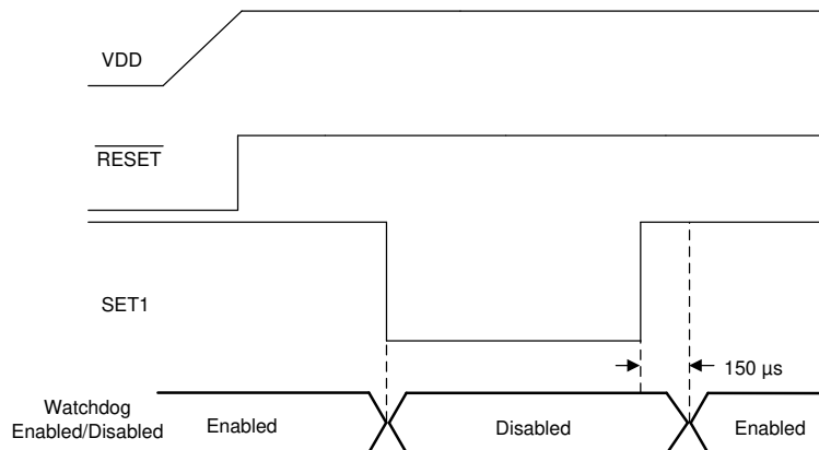
図 6-3. ウォッチドッグのイネーブル / ディスエーブル
