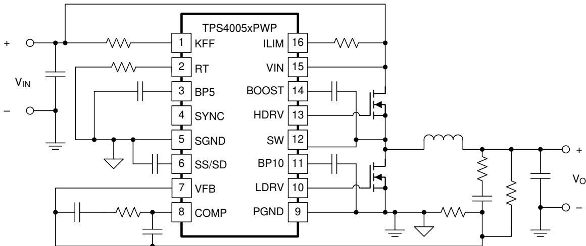
概略回路図
