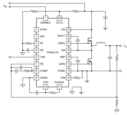
概略回路図
