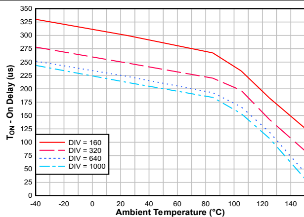
図 5-5. 入力から出力へのオン遅延 ( V_{IN} = 300\text{V} , DIV = 1000\text{V} , 双方向モード)
