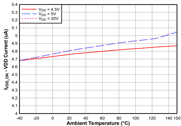
図 5-4. VDD 電流と周囲温度との関係
