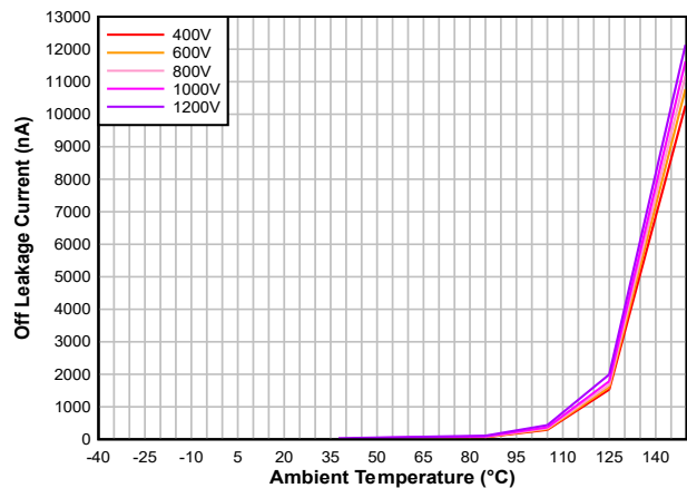
図 5-2. オフ リーク電流と周囲温度との関係
