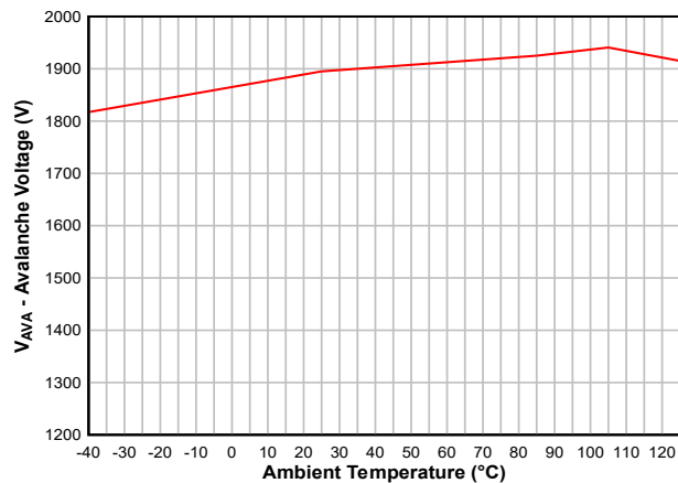
図 5-1. アバランシェ電圧と周囲温度との関係 ( I_O = 10\mu\text{A} )
