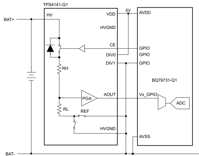
図 7-2. 単方向測定、 DIV_{NOM} = 320V/V
