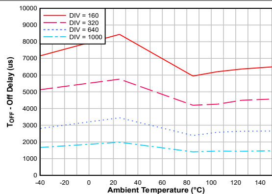
図 5-6. 入力から出力へのオフ遅延 ( V_{IN} = 300\text{V} , DIV = 1000\text{V} , 双方向モード)
