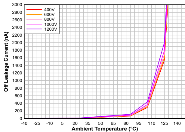
図 5-3. オフ リーク電流と周囲温度との関係 (拡大)
