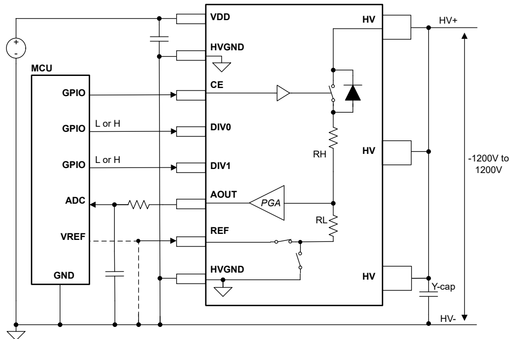
図 6-3. 双方向電圧センシング (ロジック Low または High に設定されている DIV0 および DIV1)
