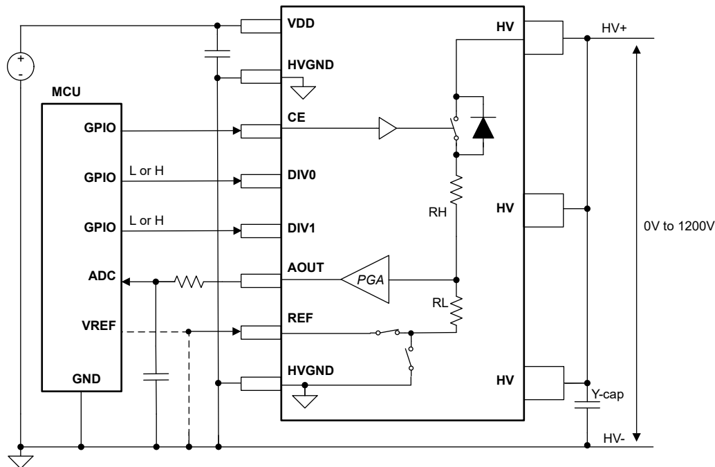
図 6-1. 単方向電圧センシング
