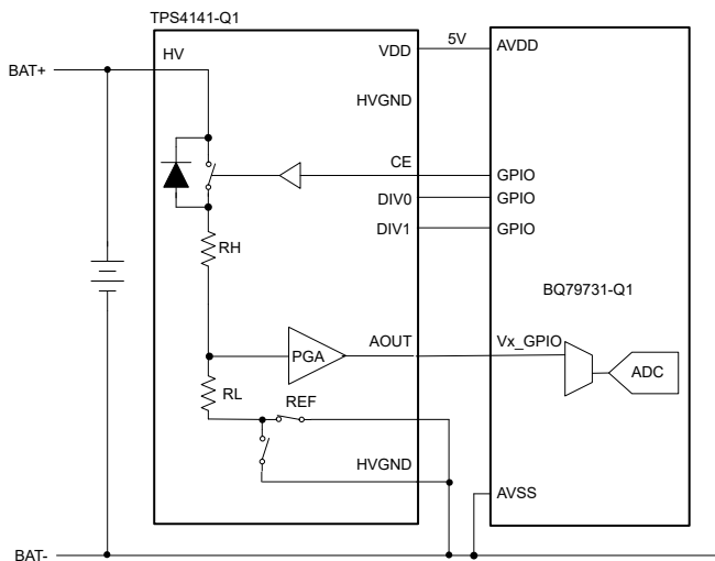
図 7-1. TPS4141-Q1 と BQ79731-Q1 を使用した DC バス測定
