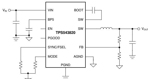
概略回路図
