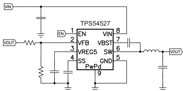
概略回路図
