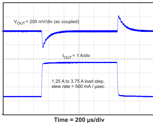
図 8-7. Transient Response
