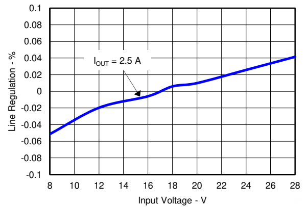
図 8-6. Line Regulation
