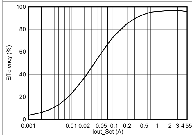
図 5-17. TPS54538 の性能 (FCCM)、 V_{IN} = 24\text{V} 、 V_{OUT} = 12\text{V} 、 f_{SW} = 500\text{kHz} 、 L = 5.6\mu\text{H}
