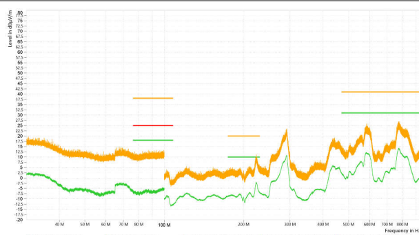
図 5-22. TPS54538、 V_{IN} = 24\text{V} 、 V_{OUT} = 5\text{V} 、 R_{OUT} = 5\text{A} 、スペクトラム拡散有効な CISPR 25 クラス 5 放射エミッション
