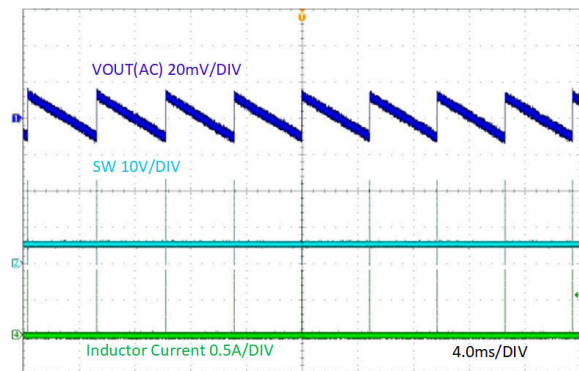
図 7-12. 定常状態、 I_{OUT} = 0A
