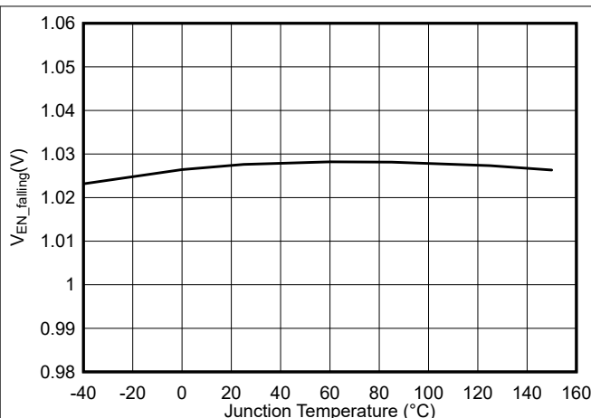
図 5-7. ディスエールスレッシュヨルドと接合部温度との関係
