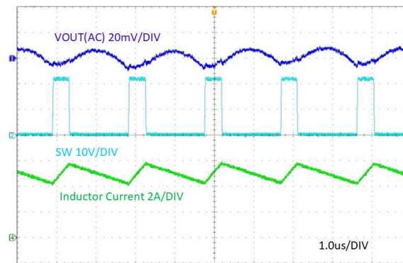
図 7-13. 定常状態、 I_{OUT} = 5A
