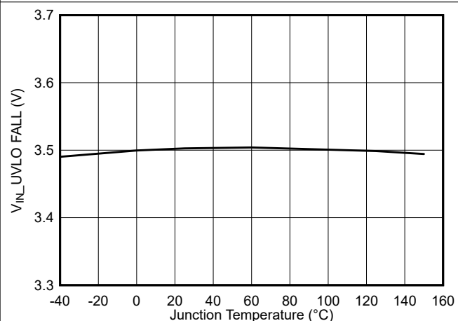
図 5-9. V_{IN} UVLO 立ち下がりスレッシュヨルド対接合部温度との関係
