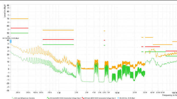
図 5-21. TPS54538、 V_{IN} = 24\text{V} 、 V_{OUT} = 5\text{V} 、 R_{OUT} = 5\text{A} 、スペクトラム拡散有効な CISPR 25 クラス 5 伝導エミッション
