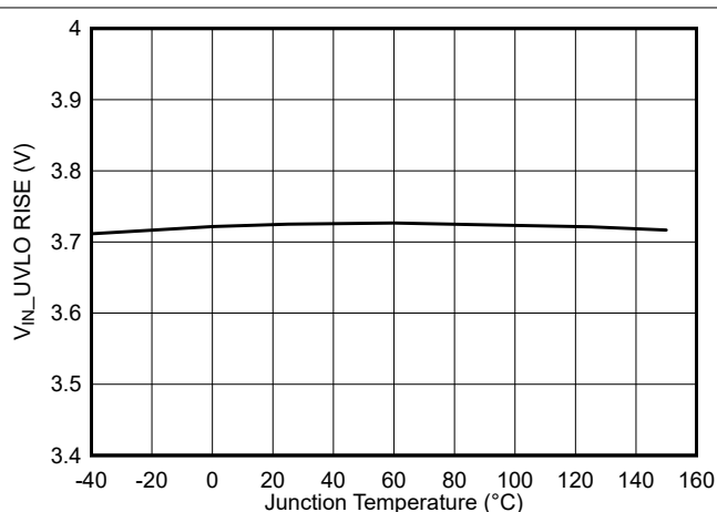
図 5-8. V_{IN} UVLO 立ち上がりスレッシュヨルド対接合部温度との関係
