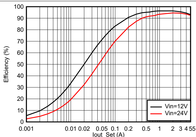
図 7-3. 効率 (FCCM)
