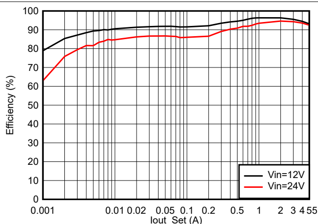
図 7-2. 効率 (PFM)
