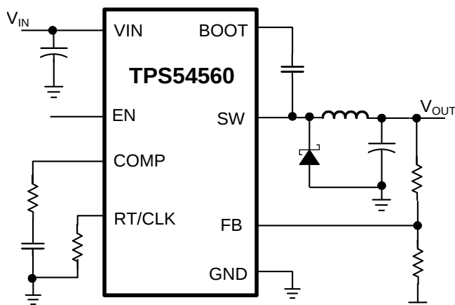
概略回路図
