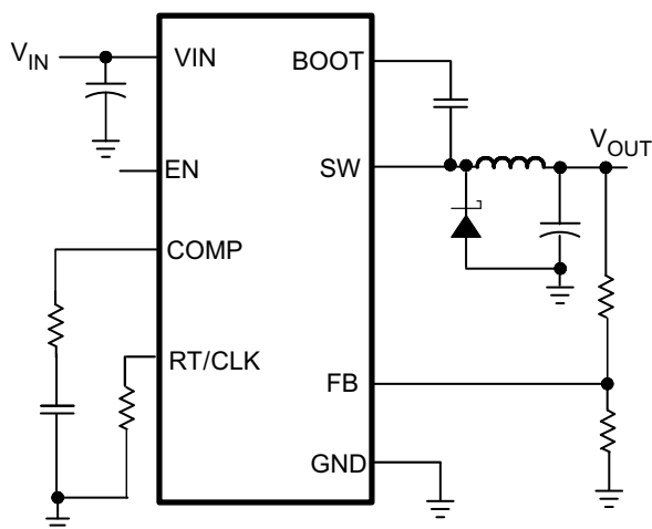
概略回路図
