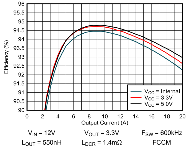
図 5-5. V_{OUT} = 3.3V での効率と V_{CC} との関係
