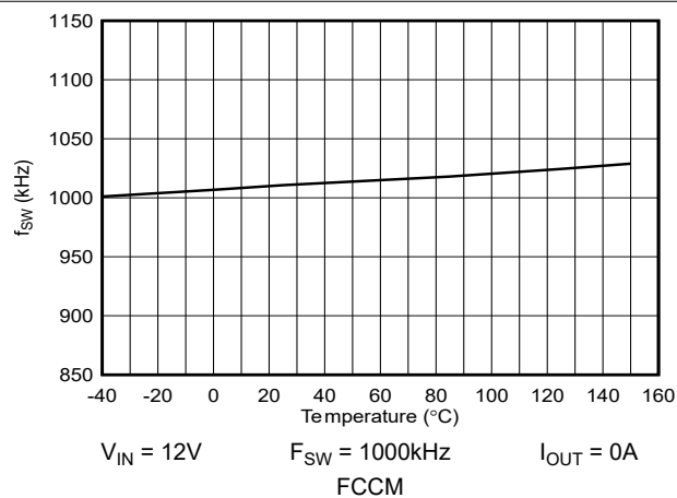
図 5-26. スイッチング周波数と接合部温度との関係
