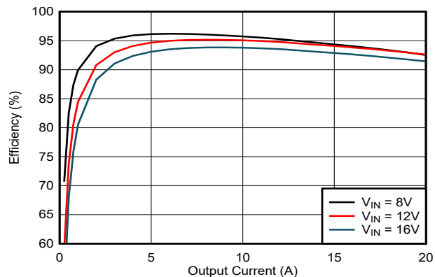
図 7-3. 効率 – FCCM モード
