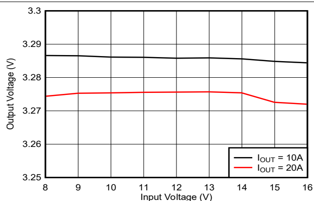
図 7-5. ラインレギュレーション
