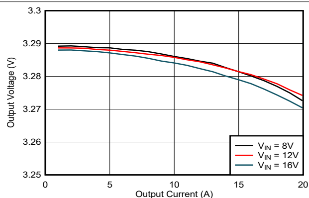
図 7-4. ロードレギュレーション
