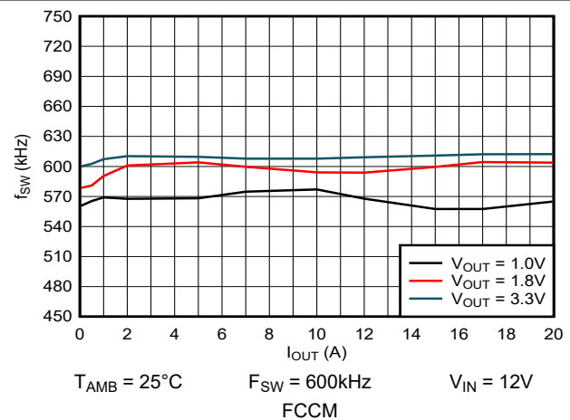
図 5-22. スイッチング周波数 対 出力電流
