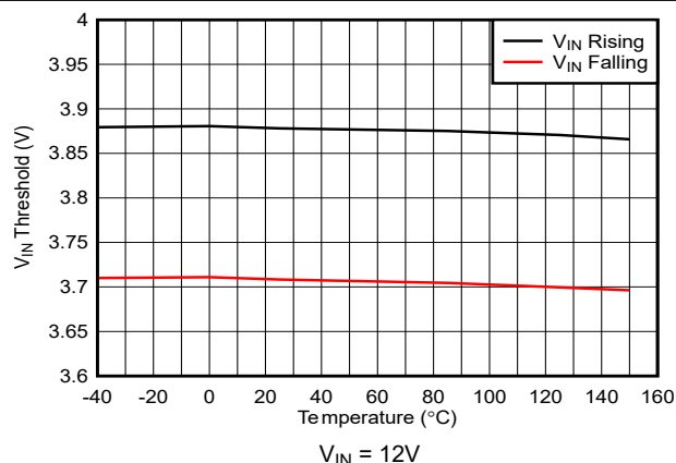
図 5-11. V_{IN} ピン低電圧誤動作防止と接合部温度との関係
