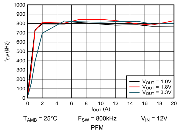
図 5-20. スイッチング周波数 対 出力電流
