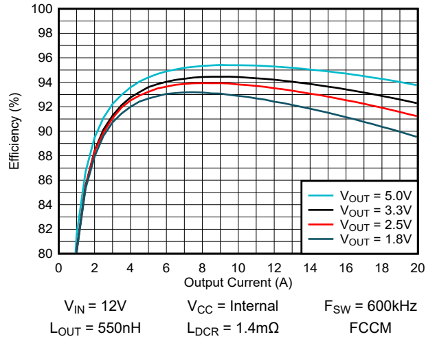
図 5-1. V_{OUT} \geq 1.8V での効率
