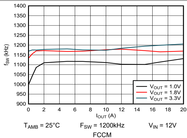
図 5-16. スイッチング周波数 対 出力電流
