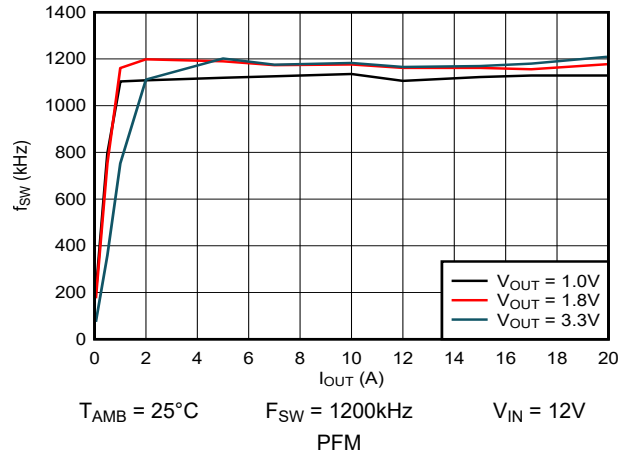
図 5-17. スイッチング周波数 対 出力電流
