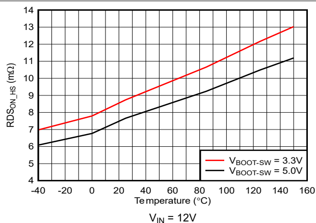
図 5-28. R_{DS(on)(HS)} と接合部温度との関係
