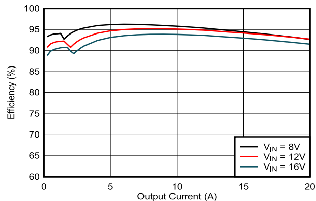
図 7-2. 効率 – PFM モード
