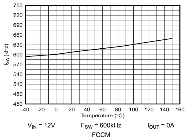
図 5-24. スイッチング周波数と接合部温度との関係
