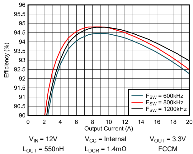
図 5-3. V_{OUT} = 3.3V での効率と F_{SW} との関係
