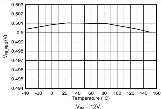
図 5-12. V_{FB\_REG} と接合部温度との関係
