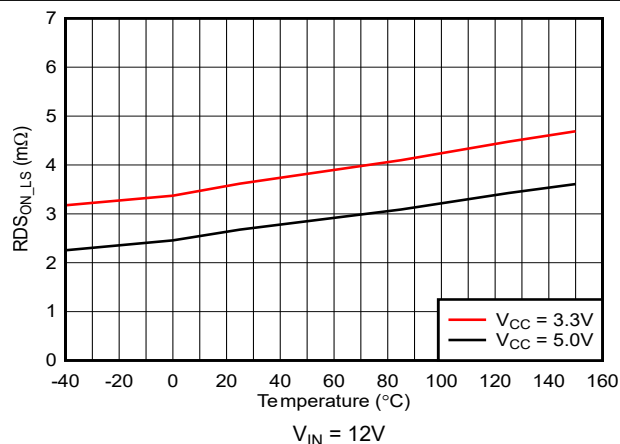
図 5-29. R_{DS(on)} と接合部温度との関係
