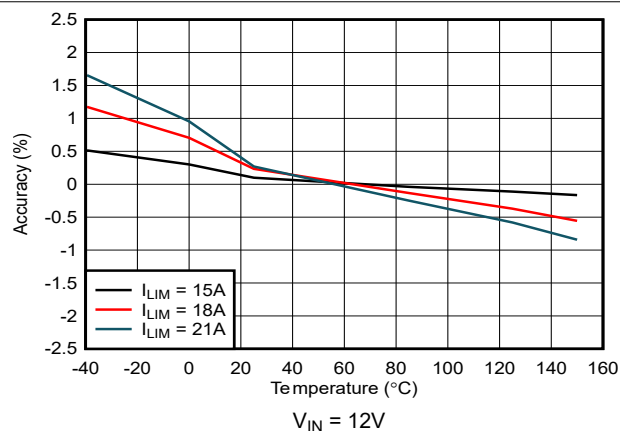
図 5-31. ローサイドバレー電流制限精度 (外部) と接合部温度との関係
