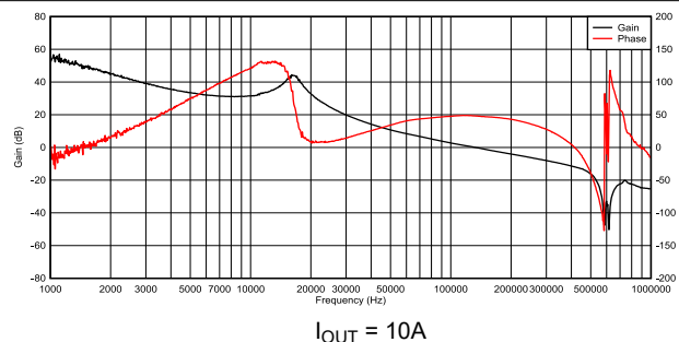
図 7-7. 周波数応答
