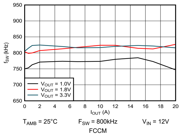
図 5-19. スイッチング周波数 対 出力電流
