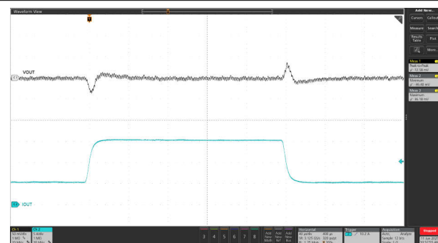
図 7-4. ロードレギュレーション
