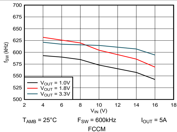
図 5-21. スイッチング周波数と入力電圧との関係
