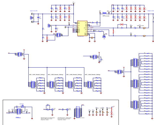
図 7-1. アプリケーション回路図
