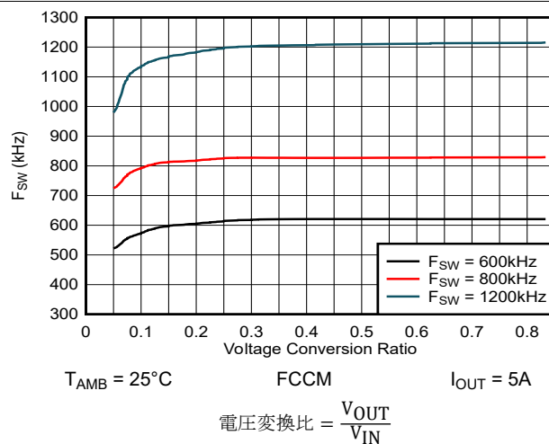
図 5-14. スイッチング周波数と電圧変換比との関係
