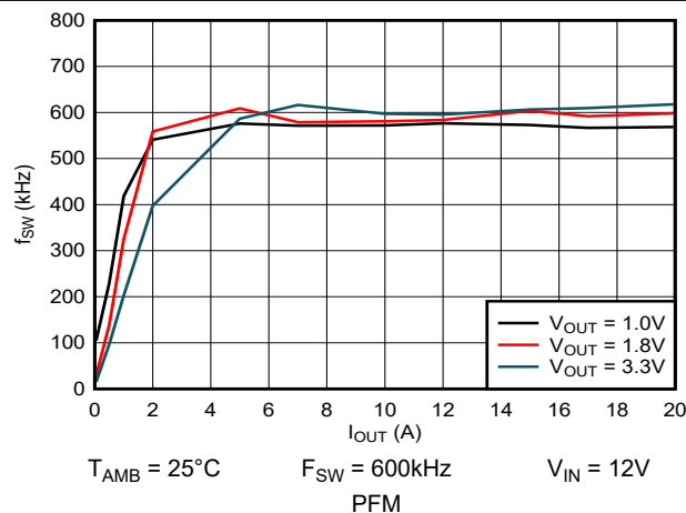
図 5-23. スイッチング周波数 対 出力電流
