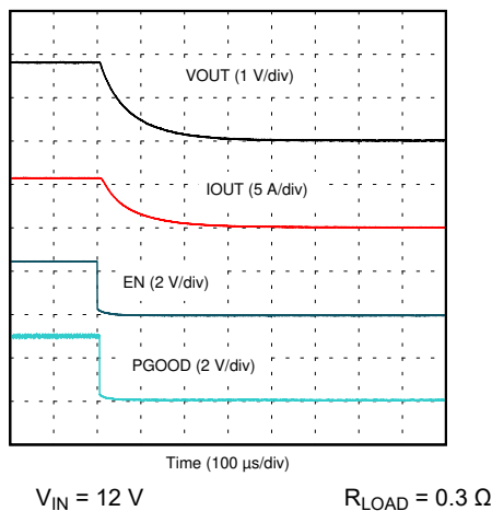
図 7-18. EN Shutdown
