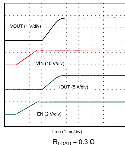
図 7-19. V_{IN} Start-Up
