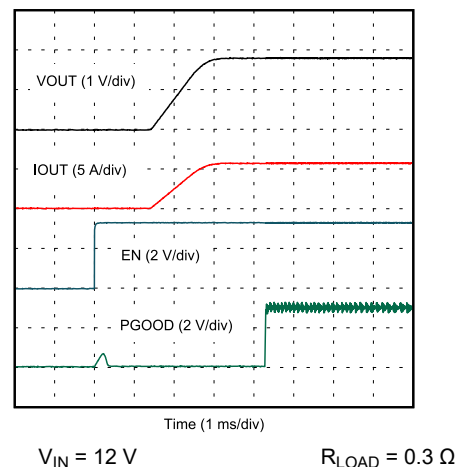
図 7-15. EN Start-Up
