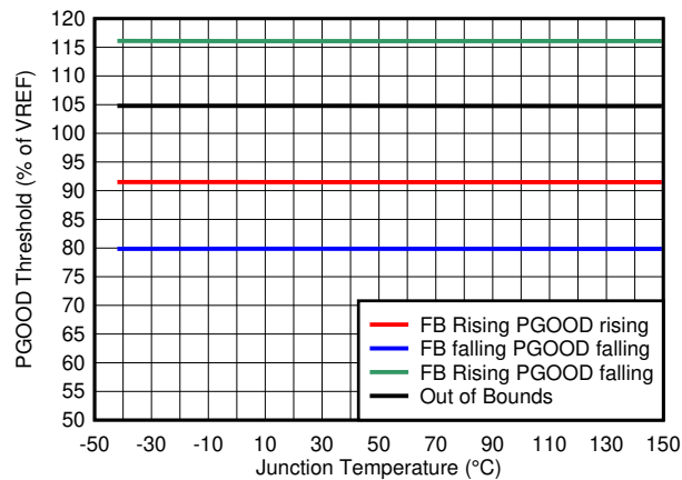
図 5-9. PGOOD Thresholds
