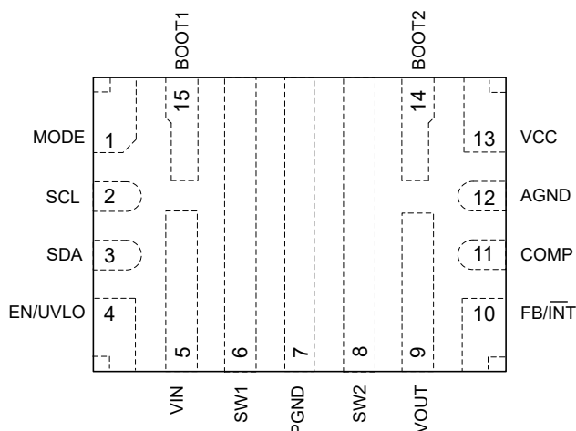
図 4-1. TPS55285A VAL パッケージ、15 ピン WQFN-HR (透過上面図)
