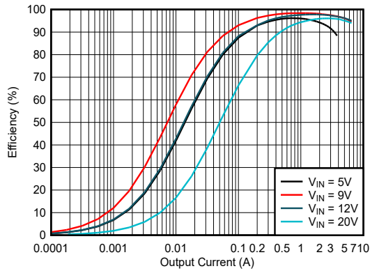
図 5-3. 効率と出力電流との関係、 V_{OUT} = 9V , FPWM
