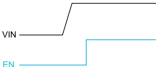
図 6-3. パワーアップ シーケンシング要件
