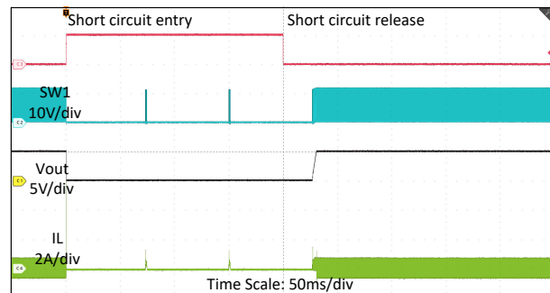
図 8-14. V_{IN} = 12V 、 V_{OUT} = 5V 、 I_{OUT} = 0.1A における短絡保護回路
