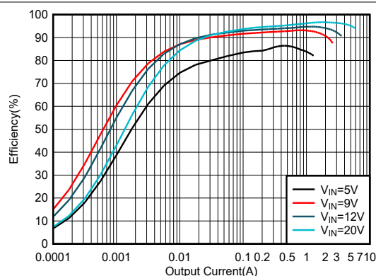
図 5-10. 効率と出力電流との関係、 V_{OUT} = 20V , PFM
