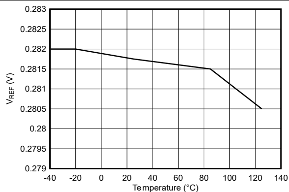
図 5-11. リファレンス電圧と温度との関係 ( V_{REF} = 0.282V )
