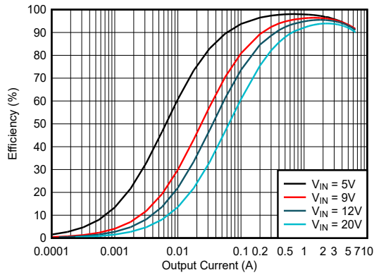
図 5-1. 効率と出力電流との関係、 V_{OUT} = 5V , FPWM
