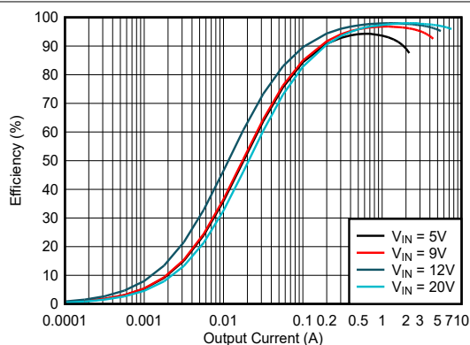
図 5-7. 効率と出力電流との関係、 V_{OUT} = 15V , FPM
