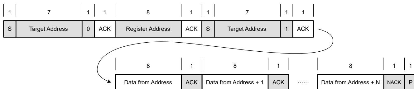
図 6-13. マルチ バイトの読み取り
