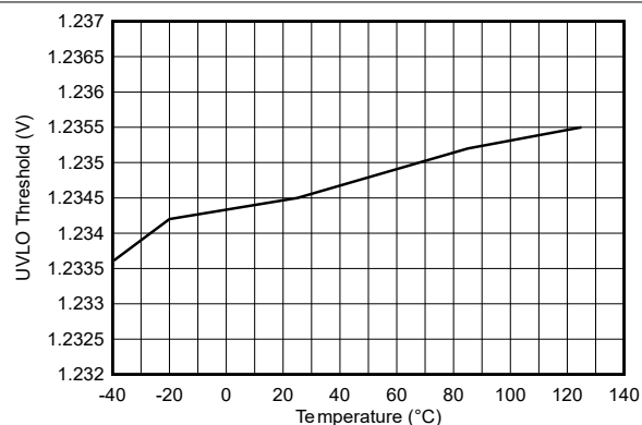
図 5-14. ENABLE/UVLO 立ち上がりスレッショルドと温度の関係
