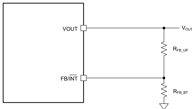
図 6-4. 外付け分圧抵抗による可変電圧設定
