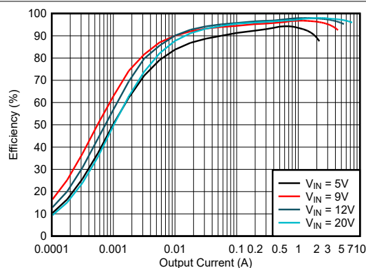
図 5-8. 効率と出力電流との関係、 V_{OUT} = 15V , PFM
