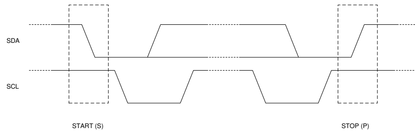
図 6-7. I²C の START 条件と STOP 条件
