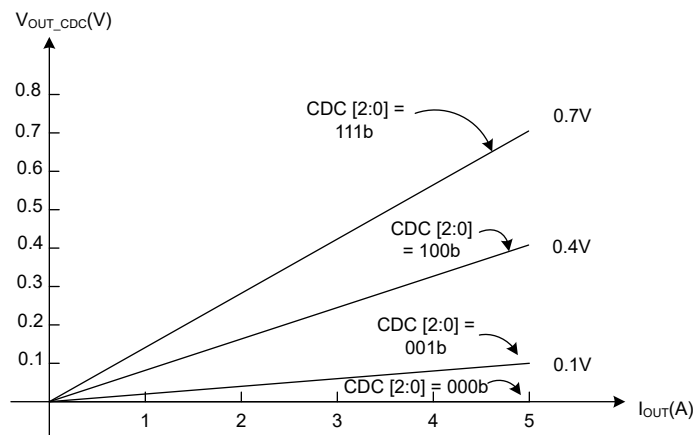
図 6-5. 出力電圧立ち上がりと出力電流との関係
