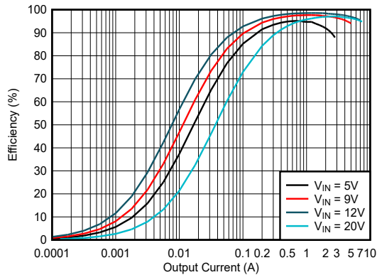
図 5-5. 効率と出力電流との関係、 V_{OUT} = 12V , FPWM
