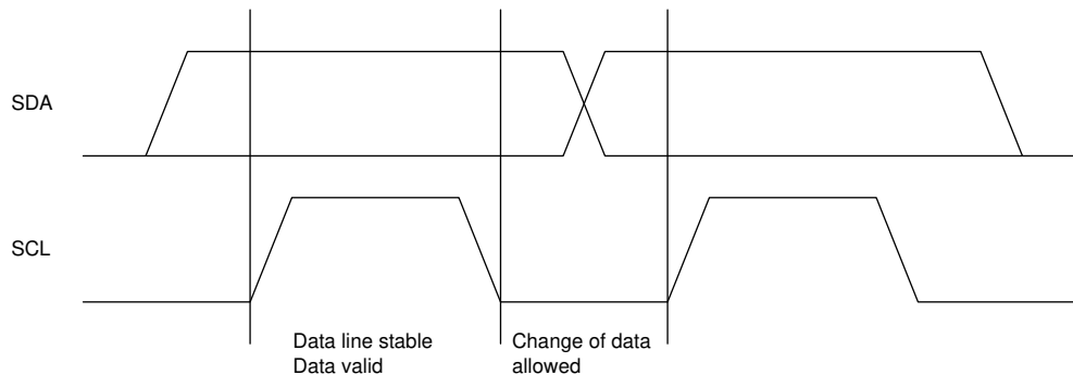
図 6-6. I 2 C データの有効性
