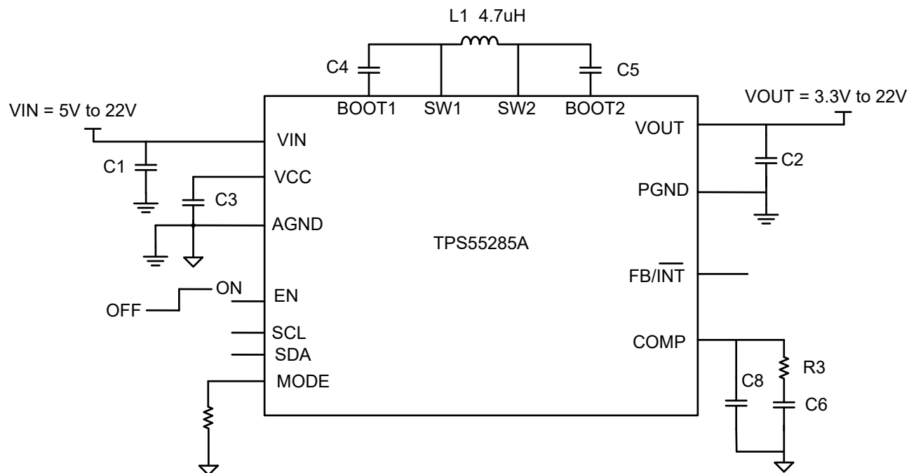
図 8-1. 電源、入力電圧 5V ~ 22V
