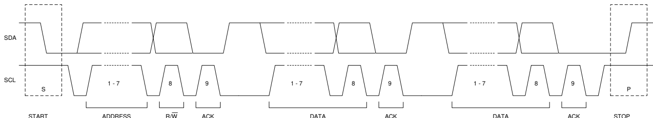
図 6-9. ターゲット アドレスとデータ方向
