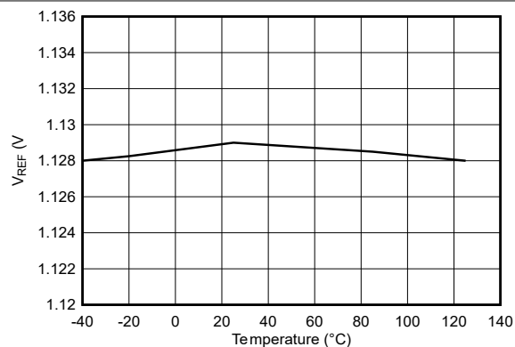
図 5-12. リファレンス電圧と温度との関係 ( V_{REF} = 1.129V )
