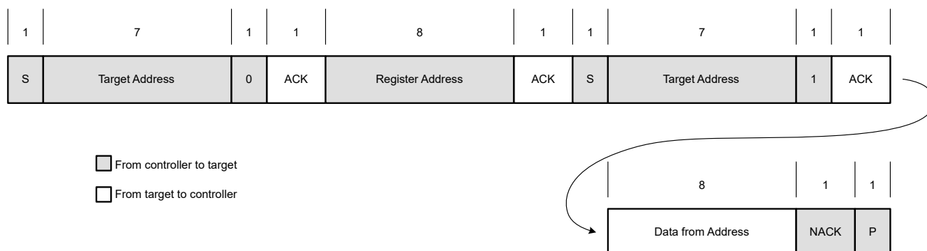
図 6-11. シングル バイトの読み取り
