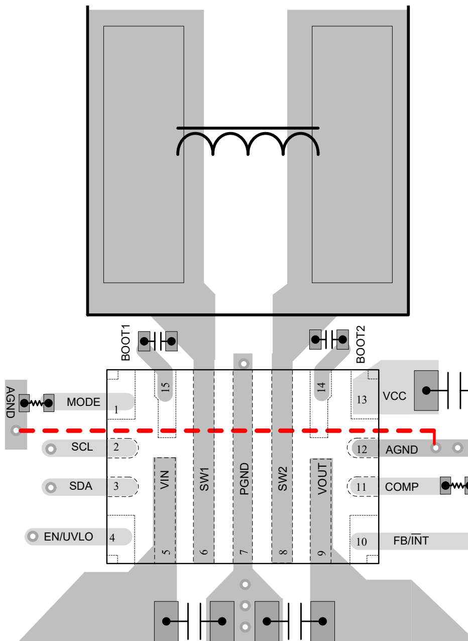
図 8-16. レイアウト例
