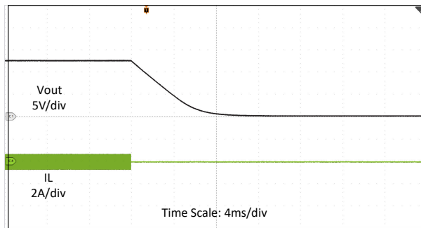
図 8-15. V_{IN} = 12V 、 V_{OUT} = 5V 、 I_{OUT} = 0A における出力放電
