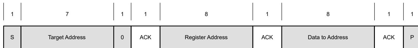
図 6-10. シングル バイトの書き込み
