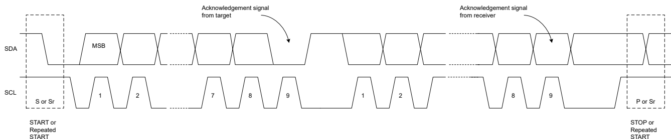
図 6-8. バイト フォーマット
