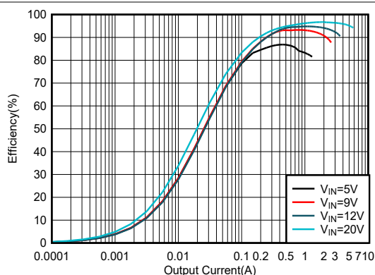
図 5-9. 効率と出力電流との関係、 V_{OUT} = 20V , FPM
