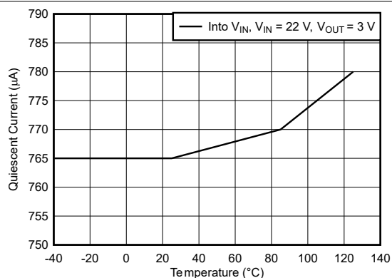
図 5-13. 静止電流と温度との関係
