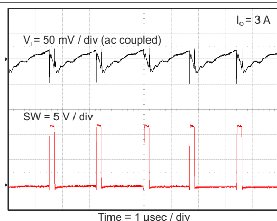
图 8-22. Tps563200 Input Voltage Ripple
