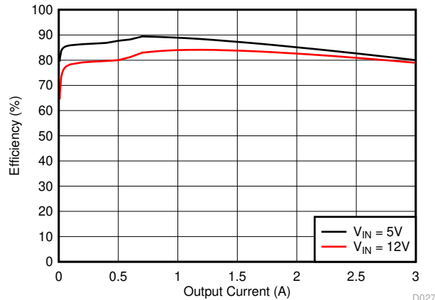
图 8-17. Tps563200 Efficiency
