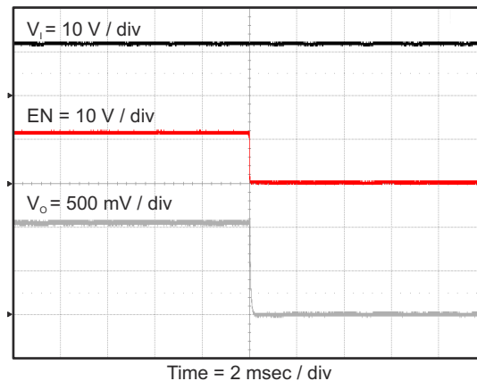
図 8-15. Tps562200 Shut Down Relative to En
