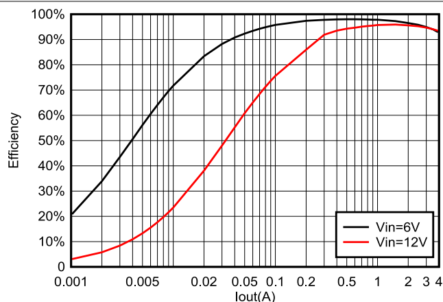
図 5-20. 4.7µH インダクタでの 5V OUT での TPS564257B の効率
