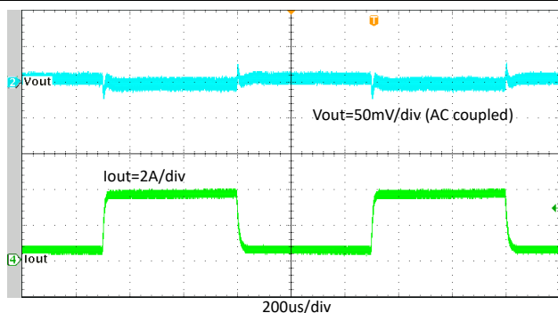
図 7-16. TPS564257B 0.4A～3.6A での過渡応答
