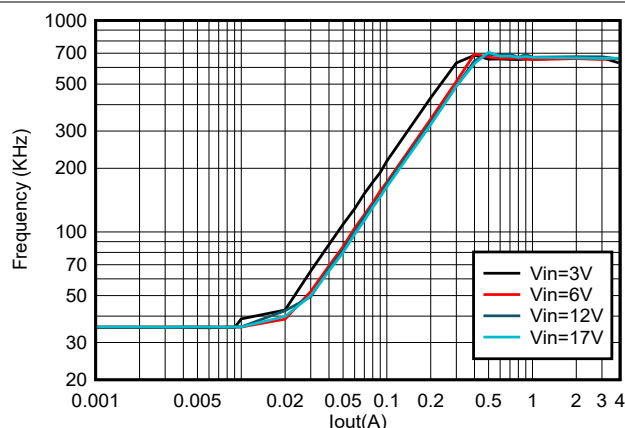
図 7-4. TPS564255B 周波数と負荷との関係
