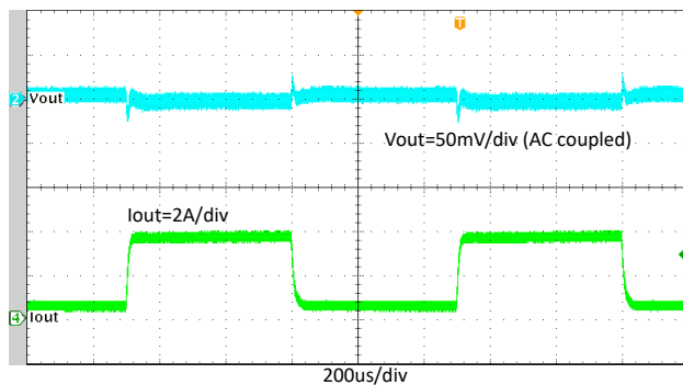
図 7-15. TPS564252B 0.4A～3.6A での過渡応答
