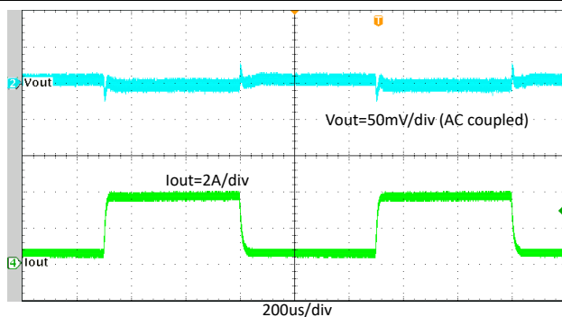
図 7-17. TPS564255B 0.4A～3.6A での過渡応答
