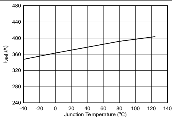
図 5-2. TPS564257B、TPS564257C の静止電流
