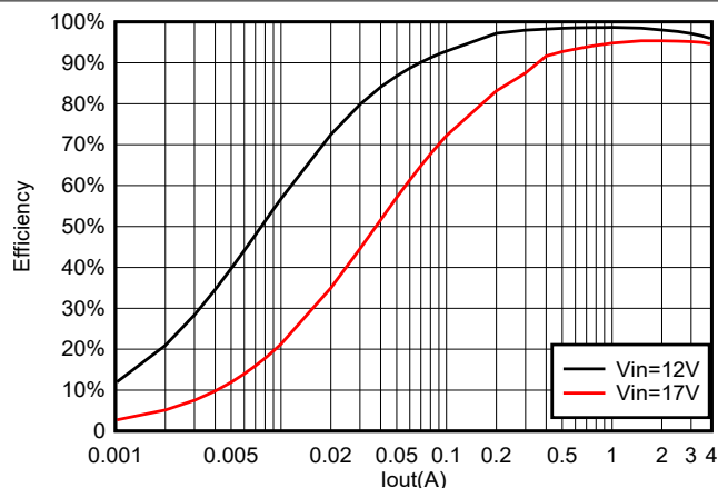
図 5-23. 6.8µH インダクタでの 10V OUT での TPS564257B の効率
