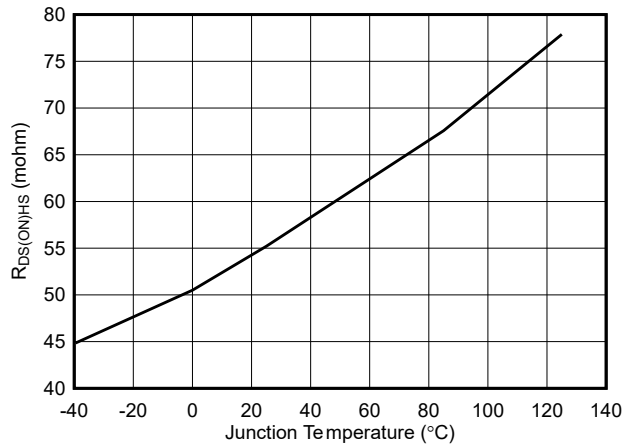
図 5-7. ハイサイド R_{DS(ON)}
