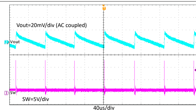
図 7-11. TPS564252B 出力電圧リップル (0.01A 負荷)
