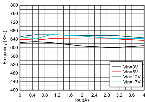
図 7-3. TPS564257B 周波数と負荷との関係
