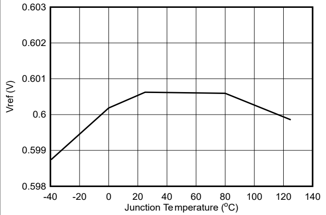
図 5-8. VREF 電圧
