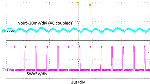
図 7-14. 出力電圧リップル (4A 負荷)
