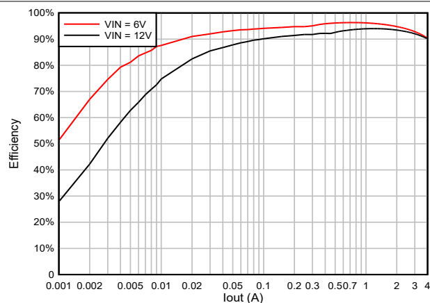
図 5-25. 2.2 \mu\text{H} インダクタでの 3.3V OUT での TPS564252C の効率
