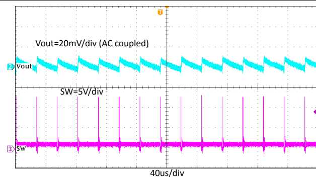
図 7-13. TPS564255B 出力電圧リップル (0.01A 負荷)
