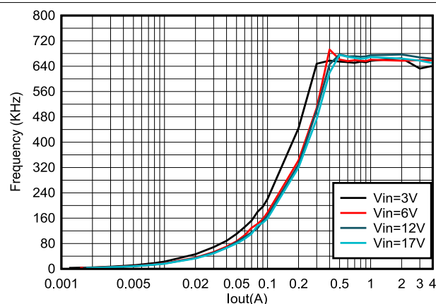
図 7-2. TPS564252B 周波数と負荷との関係
