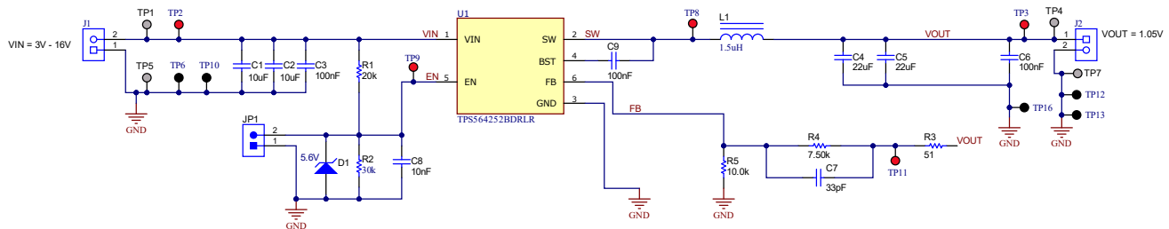
図 7-1. 回路図
