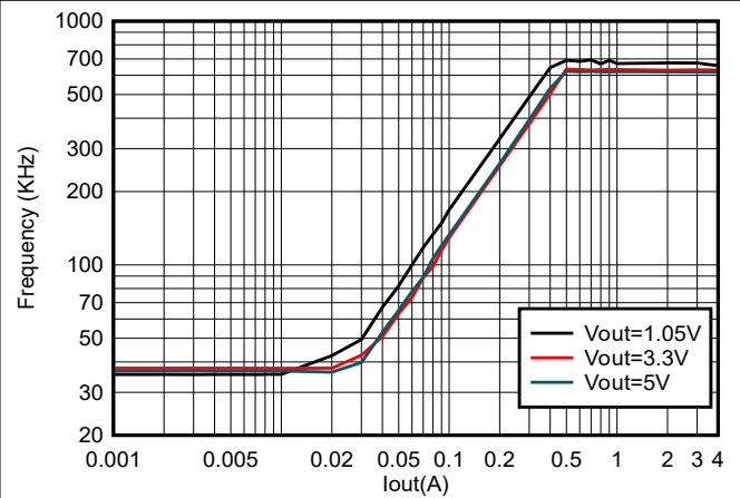
図 5-12. TPS564255B 周波数と負荷との関係 ( V_{IN} = 12\text{V} )
