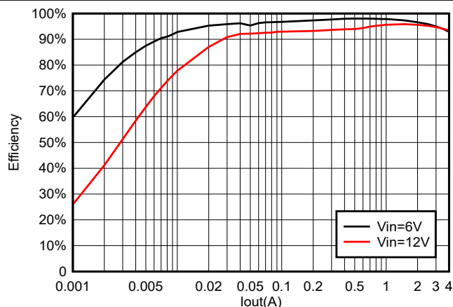
図 5-21. 4.7µH インダクタでの 5V OUT での TPS564255B の効率
