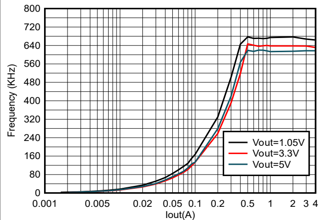
図 5-10. TPS564252B 周波数と負荷との関係 ( V_{IN} = 12\text{V} )
