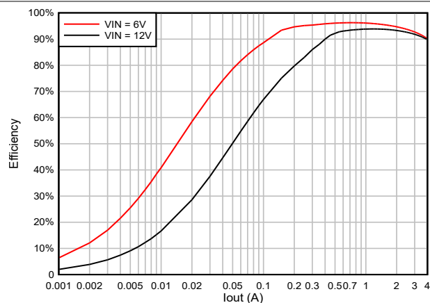
図 5-26. 2.2 \mu\text{H} インダクタでの 3.3V OUT での TPS564257C の効率
