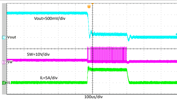
図 7-22. TPS564252B 通常動作から出力のハード短絡
