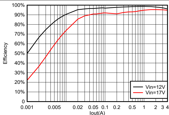
図 5-24. 6.8µH インダクタでの 10V OUT での TPS564255B の効率
