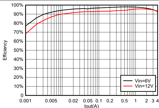
図 5-19. 4.7µH インダクタでの 5V OUT での TPS564252B の効率
