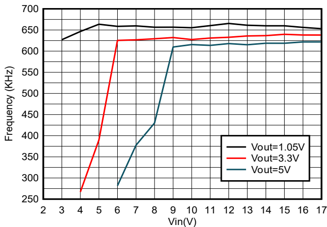
図 5-9. TPS564257B 周波数と入力電圧との関係 ( I_{OUT} = 4\text{A} )
