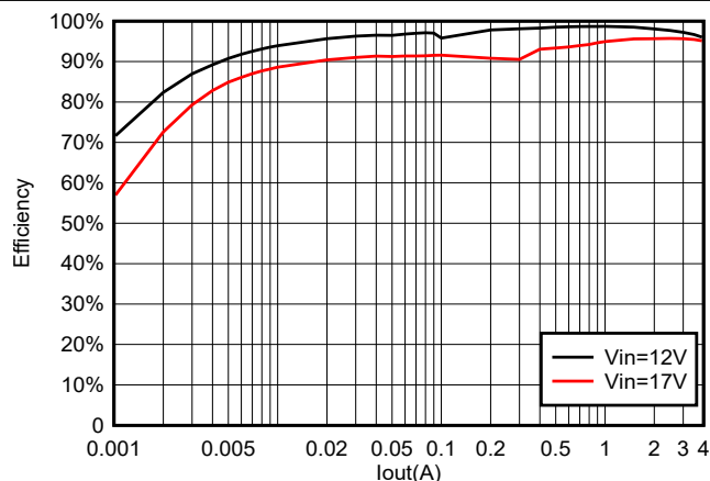
図 5-22. 6.8µH インダクタでの 10V OUT での TPS564252B の効率
