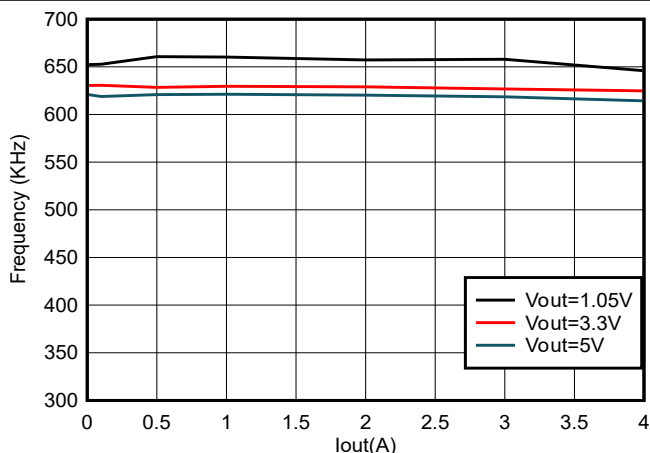
図 5-11. TPS564257B 周波数と負荷との関係 ( V_{IN} = 12\text{V} )
