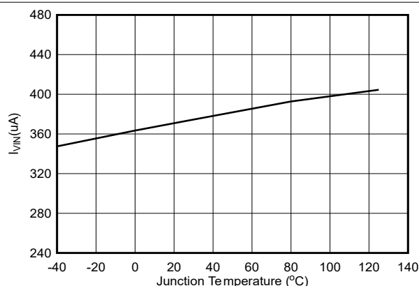
図 5-3. TPS564255B の静止電流
