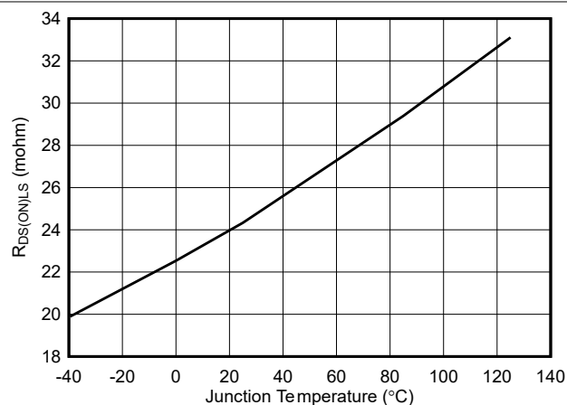
図 5-6. ローサイド R_{DS(ON)}
