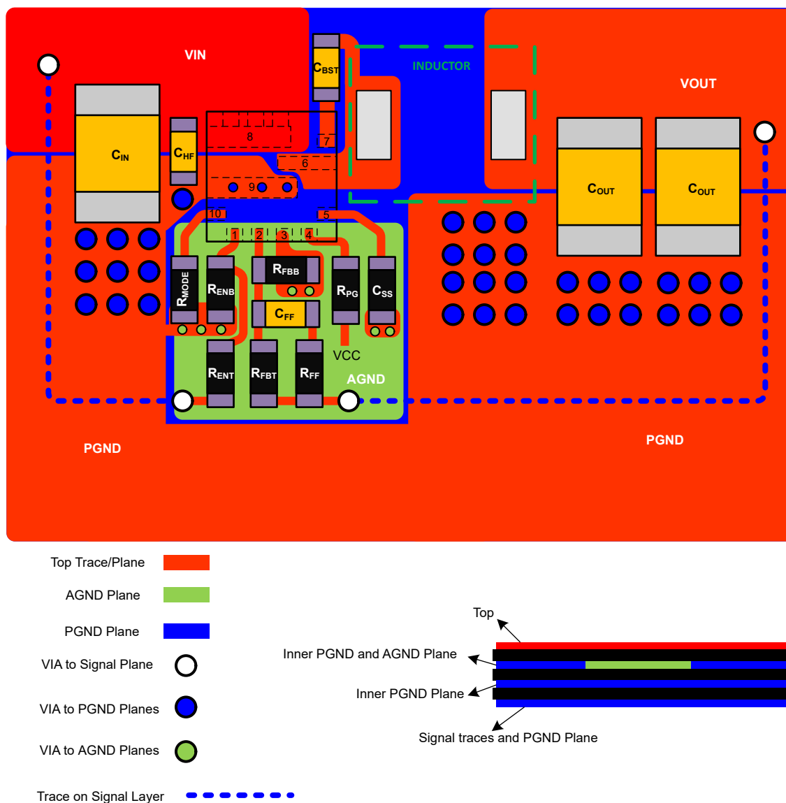
図 7-18. TPS56837 layout
