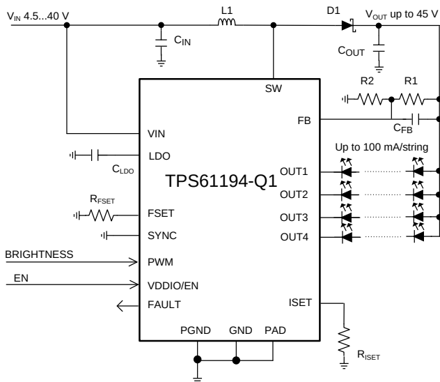
応用回路例
