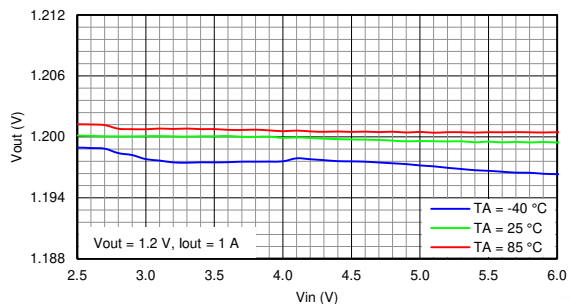
图 9-6. Line Regulation
