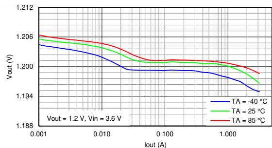
图 9-7. Load Regulation
