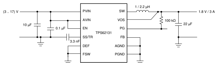
代表的なアプリケーション回路図
