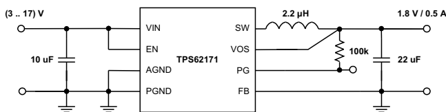
代表的なアプリケーションの回路図
