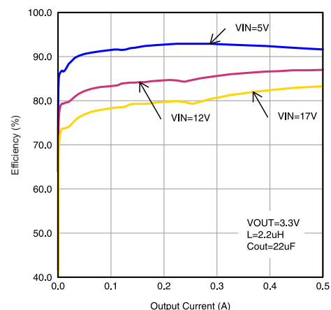
効率と出力電流との関係
