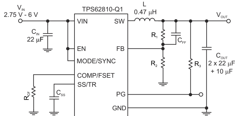
図 9-1. 代表的なアプリケーション
