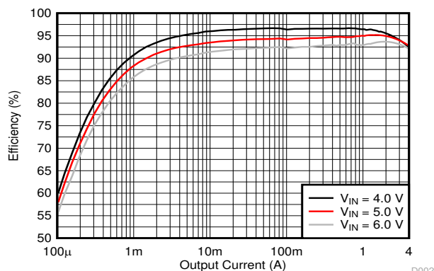
効率と出力電流との関係、 V_{OUT} = 3.3\text{V} 、PWM/PFM、 f_s = 2.25\text{MHz}
