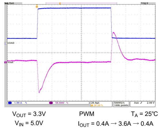
図 9-23. 負荷過渡応答
