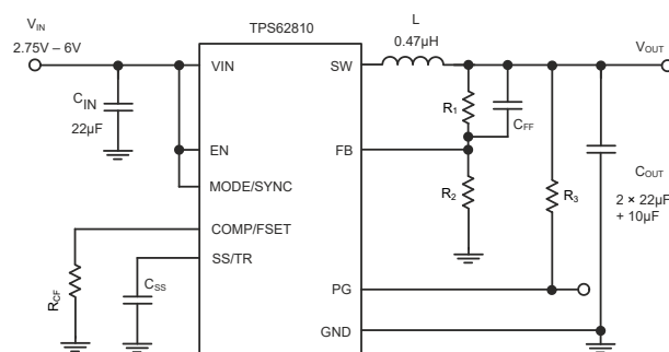
概略回路図
