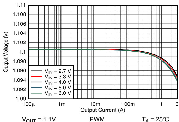
図 9-15. 出力電圧と出力電流との関係
