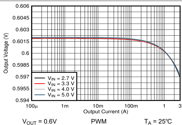
図 9-17. 出力電圧と出力電流との関係
