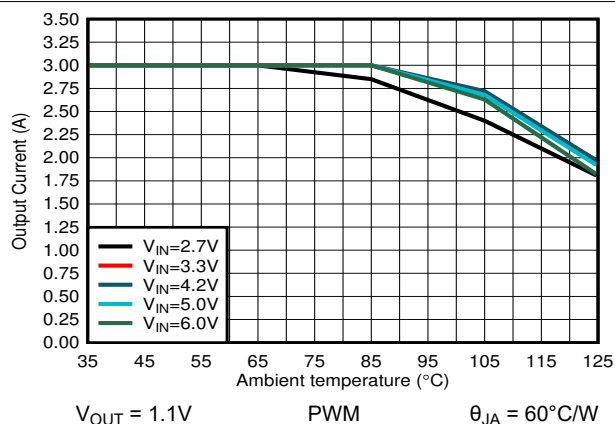
図 9-19. 出力電流と周囲温度との関係
