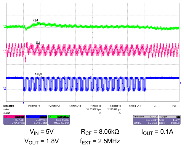
図 9-60. 外部同期から内部固定周波数へのスイッチング
