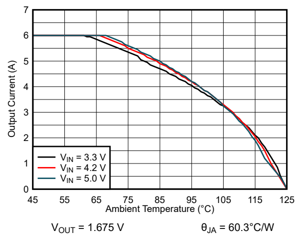
9-11. Thermal Derating
